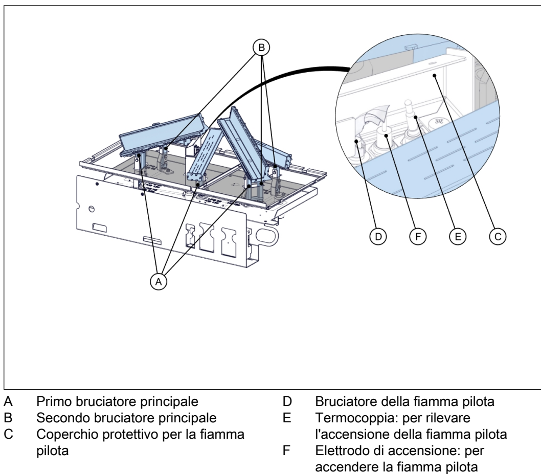
Figura 3. Alloggiamento del bruciatore e fiamma pilota
