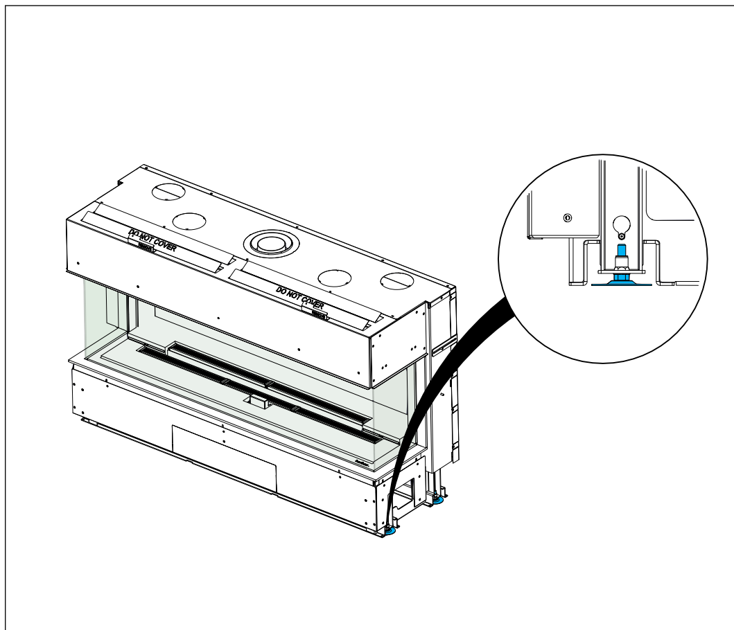
Figura 23. Alineación con los pies ajustables
