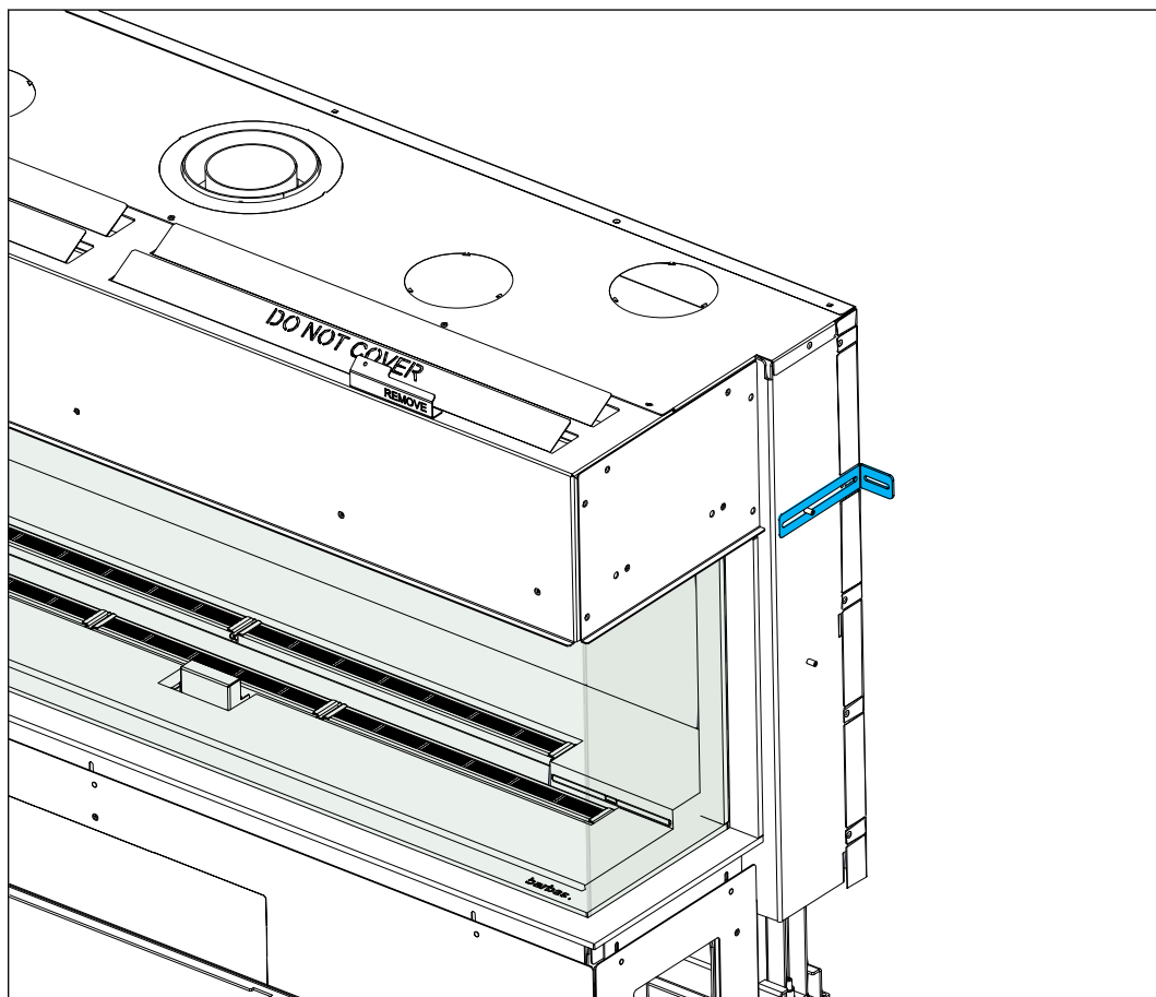
Figura 25. Fijación a la pared posterior
