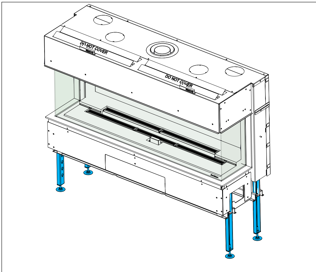
Figura 24. Alineación con patas de altura ajustable
