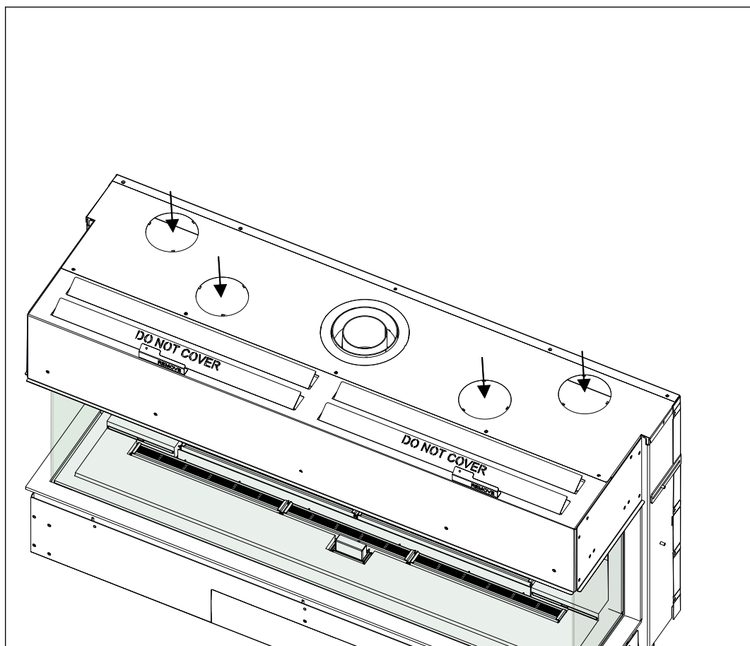
Figura 27. Posición de aberturas de salida de aire de convección
