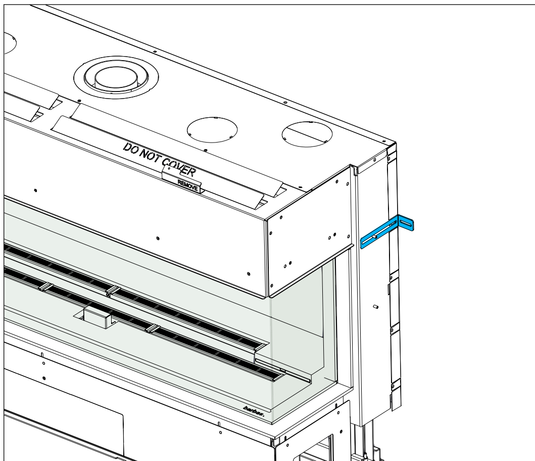
Figure 25. Fixation sur paroi arrière
