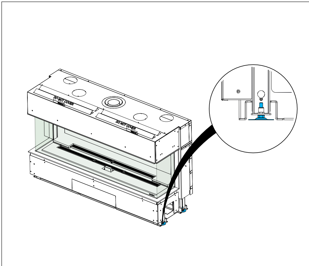
Figure 23. Alignement avec pieds réglables
