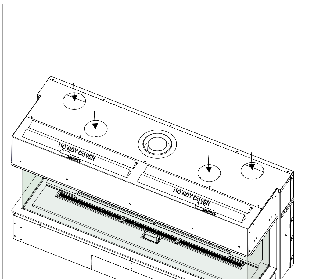
Figure 27. Position d'ouvertures de sortie d'air convection
