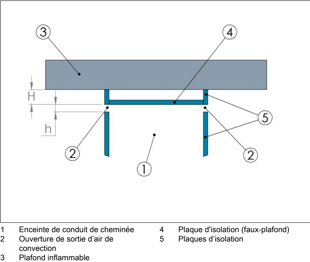
Figure 12. Dégagements avec plafond inflammable - Vue avant
