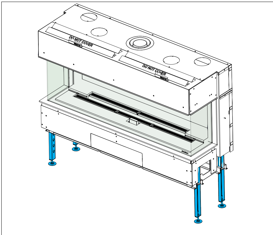
Figure 24. Alignement avec pattes réglables en hauteur
