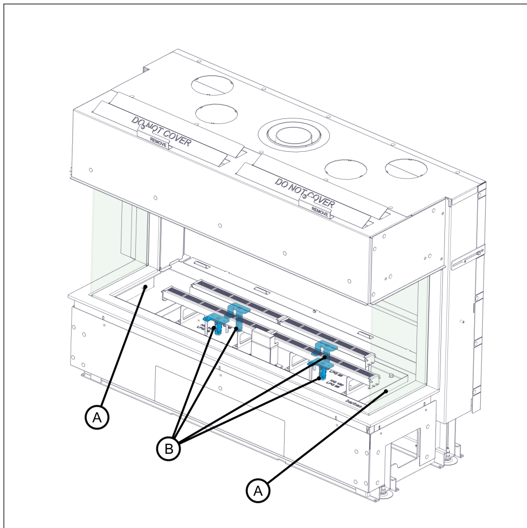
Figure 32. Positionnement des ouvertures d'entrée d'air primaire et d'admission d'air
