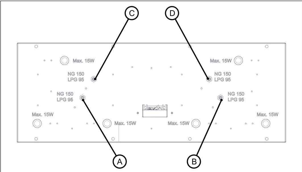
Figura 35. Posizioni degli ingressi dell'aria principali e degli iniettori di gas
