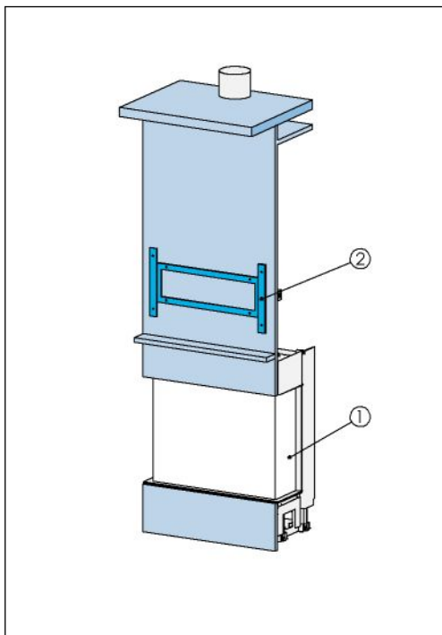
Figura 30. Installazione TV sopra all'apparecchio (vista anteriore)
