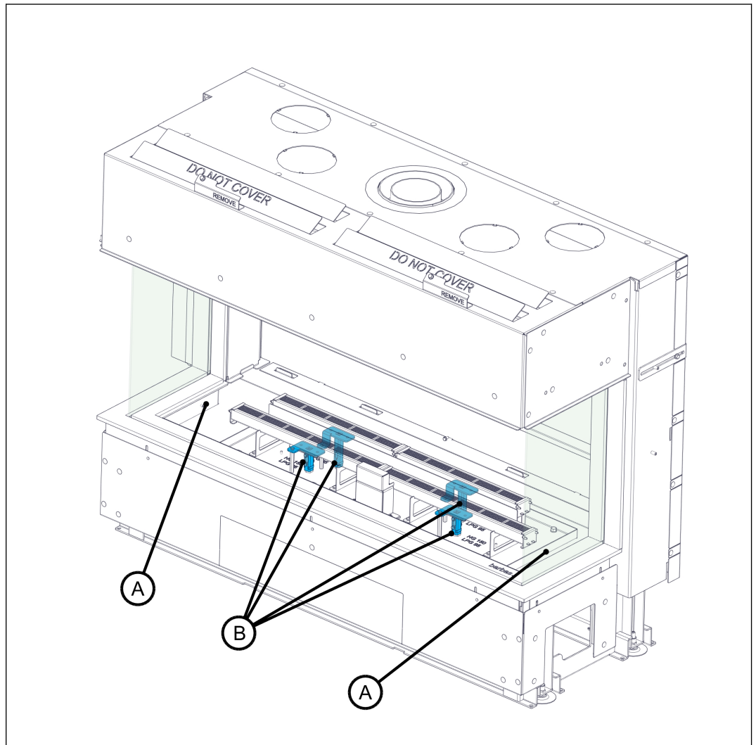
Figuur 32. Positie van luchtinlaat- en primaire luchtinlaatopeningen
