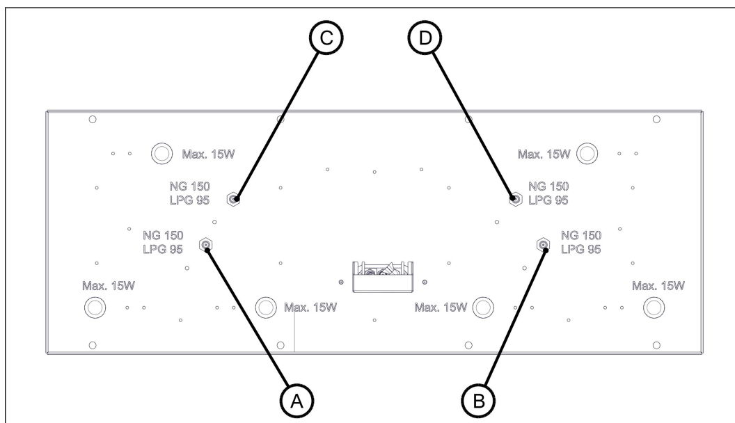
Figuur 35. Positie van primaire luchtinlaten en gasinjectoren
