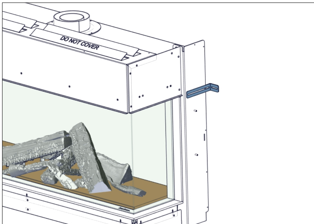
Figura 25. Fissaggio alla parete posteriore
