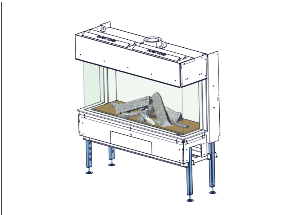
Figure 24. Alignement avec pattes réglables en hauteur
