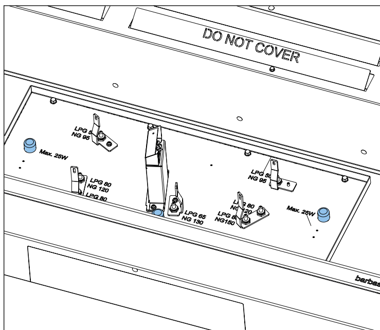
Figura 42. Posizione delle lampade per l'illuminazione ambiente
