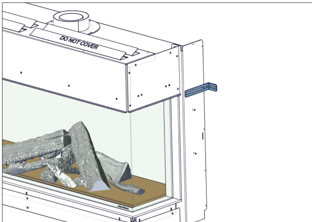
Figura 25. Fissaggio alla parete posteriore
