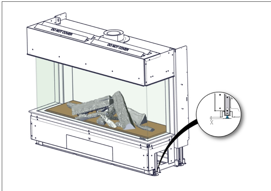
Figura 23. Allineamento con i piedini regolabili
