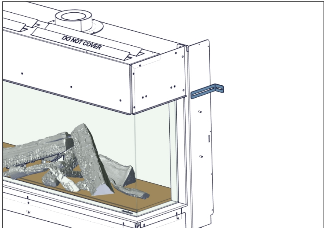
Abbildung 25. Befestigung an der Rückwand
