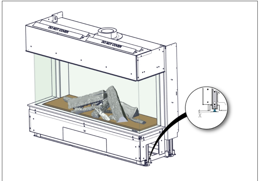
Abbildung 23. Ausrichtung mit Stellfüßen
