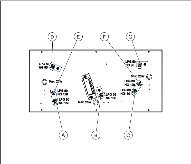
Abbildung 45. Positionen der Primärlufteinlässe und Gasinjektoren
