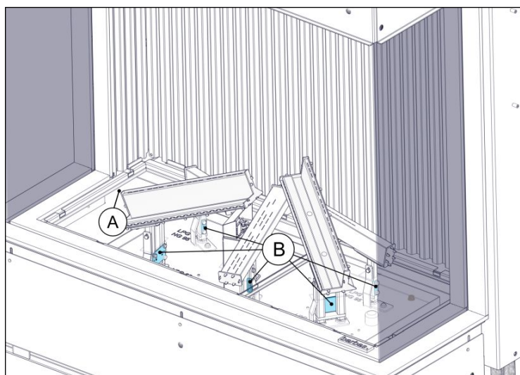
Abbildung 40. Positionen der Lufteinlass- und Primärlufteinlassöffnungen
