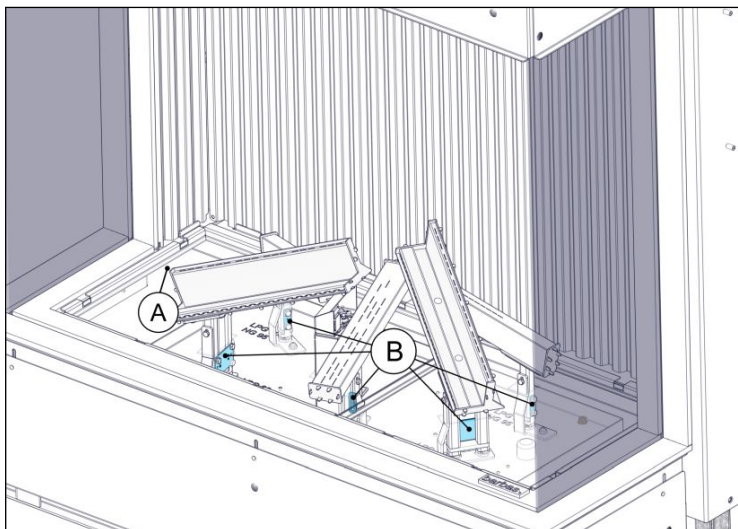
Figuur 40. Positie van luchtinlaat- en primaire luchtinlaatopeningen
