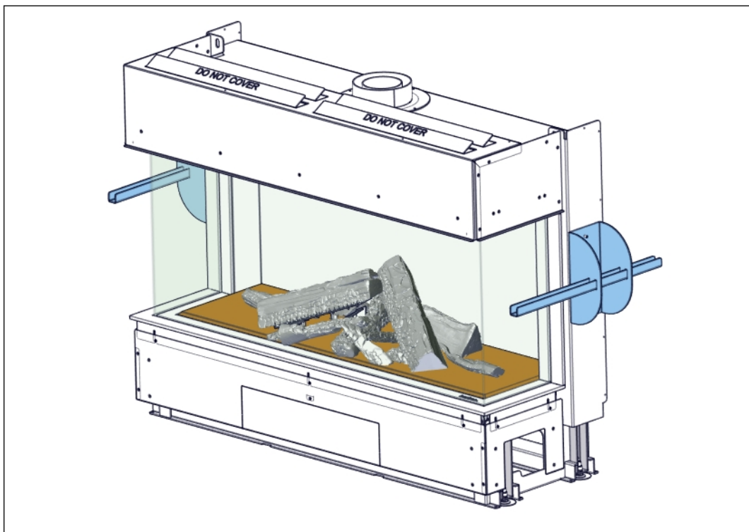
Figuur 22. Toestel met draaggrepen
