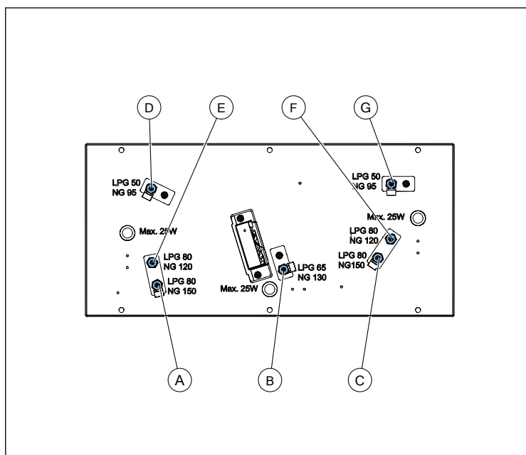
Figuur 43. Positie van primaire luchtinlaten en gasinjectoren
