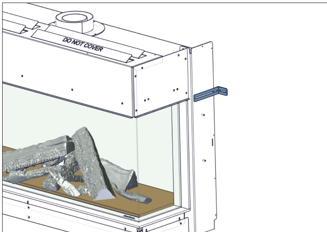
Figuur 25. Bevestiging aan de achterwand
