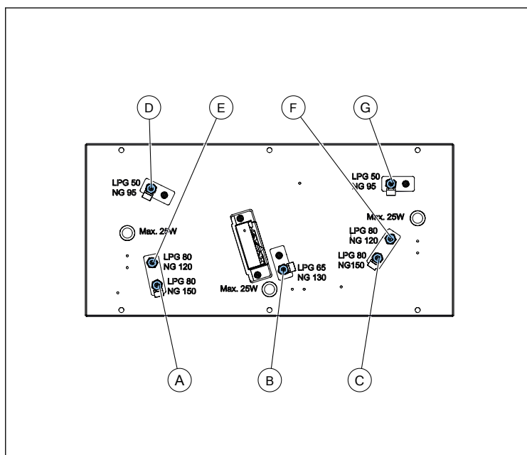
Figuur 44. Positie van primaire luchtinlaten en gasinjectoren
