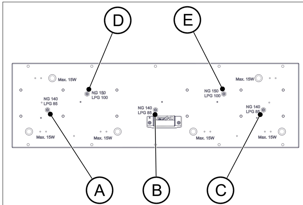
Abbildung 37. Positionen der Primärlufteinlässe und Gasinjektoren
