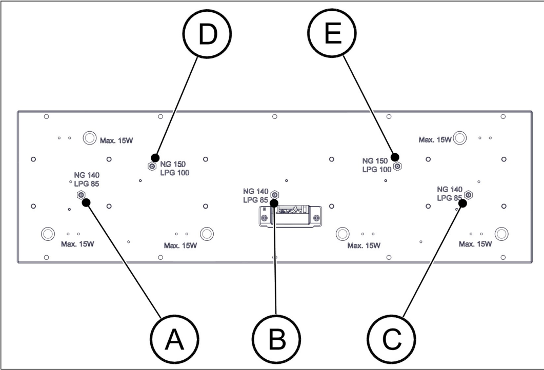
Abbildung 36. Positionen der Primärlufteinlässe und Gasinjektoren
