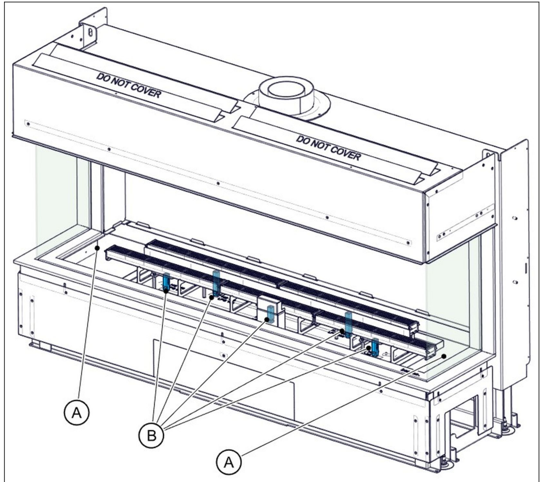
Abbildung 32. Positionen der Lufteinlass- und Primärlufteinlassöffnungen
