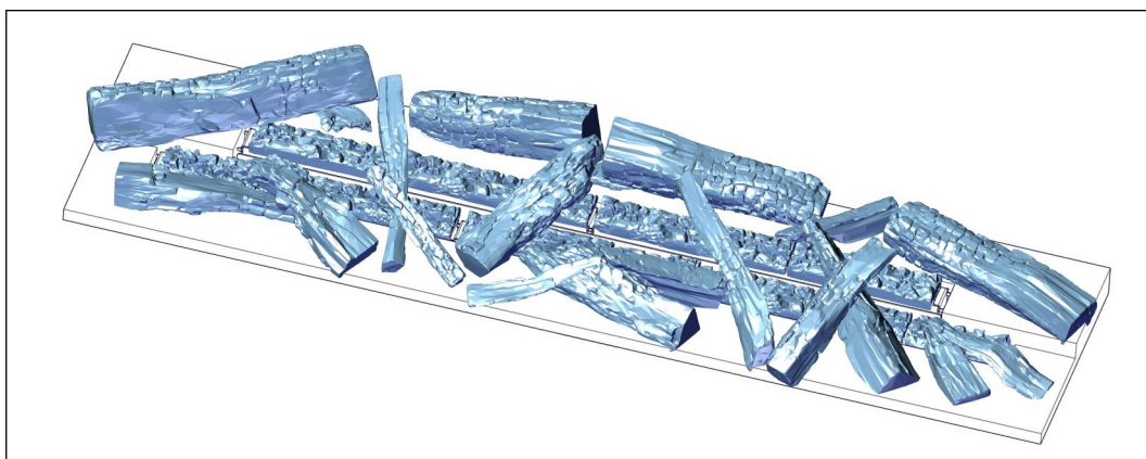
Figura 33. Posición de los troncos de madera cerámica y los quemadores
