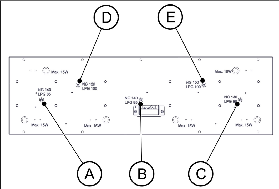
Figura 35. Posición de las entradas de aire principales y los inyectores de gas
