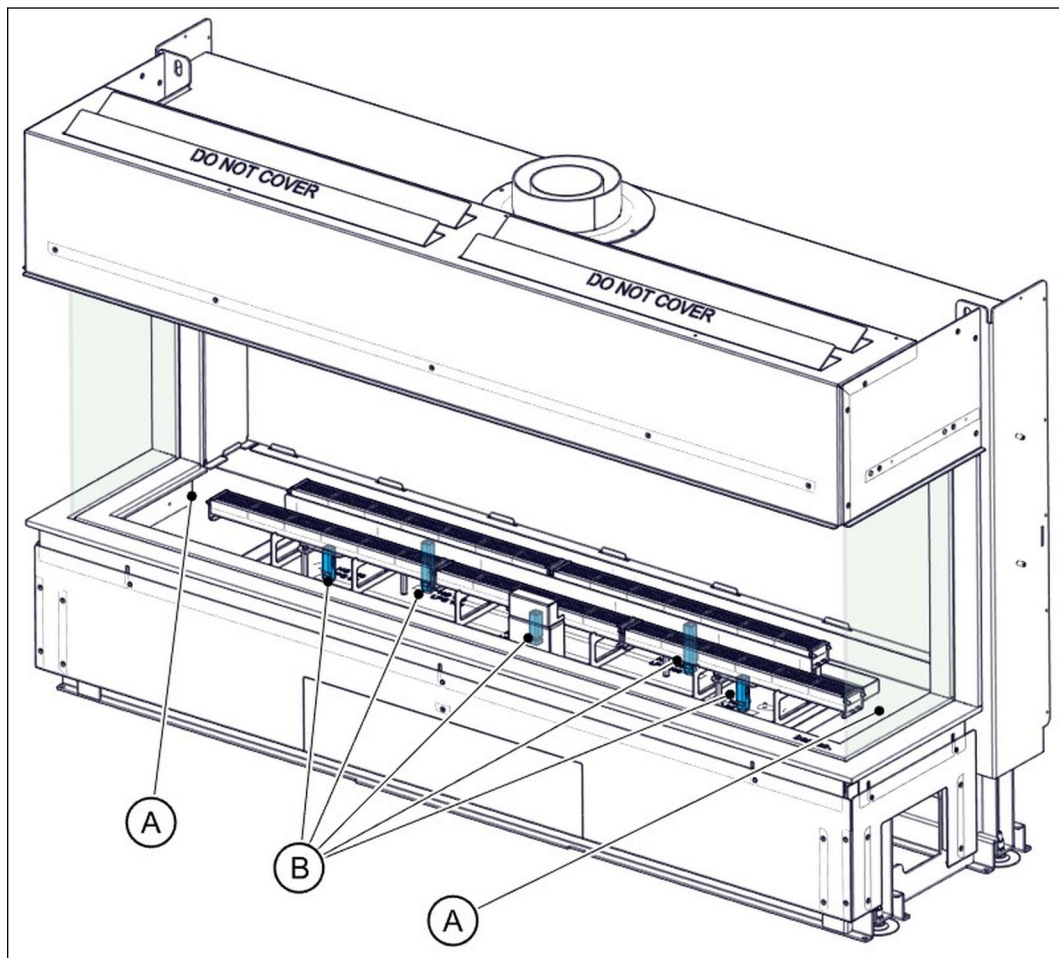
Figura 32. Posición de la entrada de aire y las aberturas de entrada de aire principales
