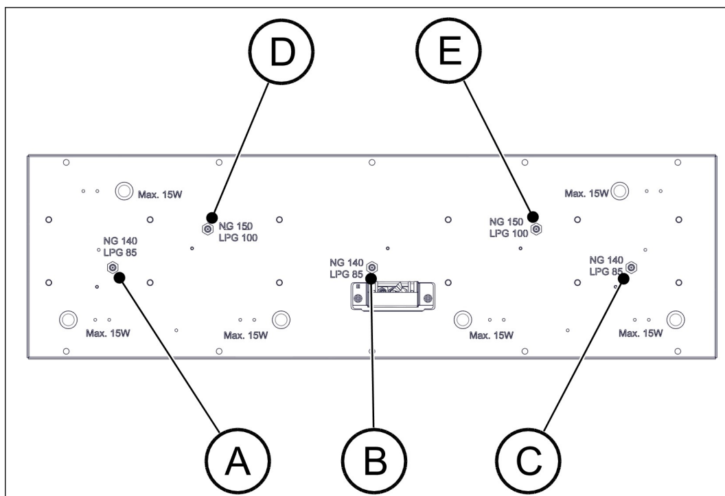
Figure 35. Position des entrées d'air primaires et des injecteurs de gaz
