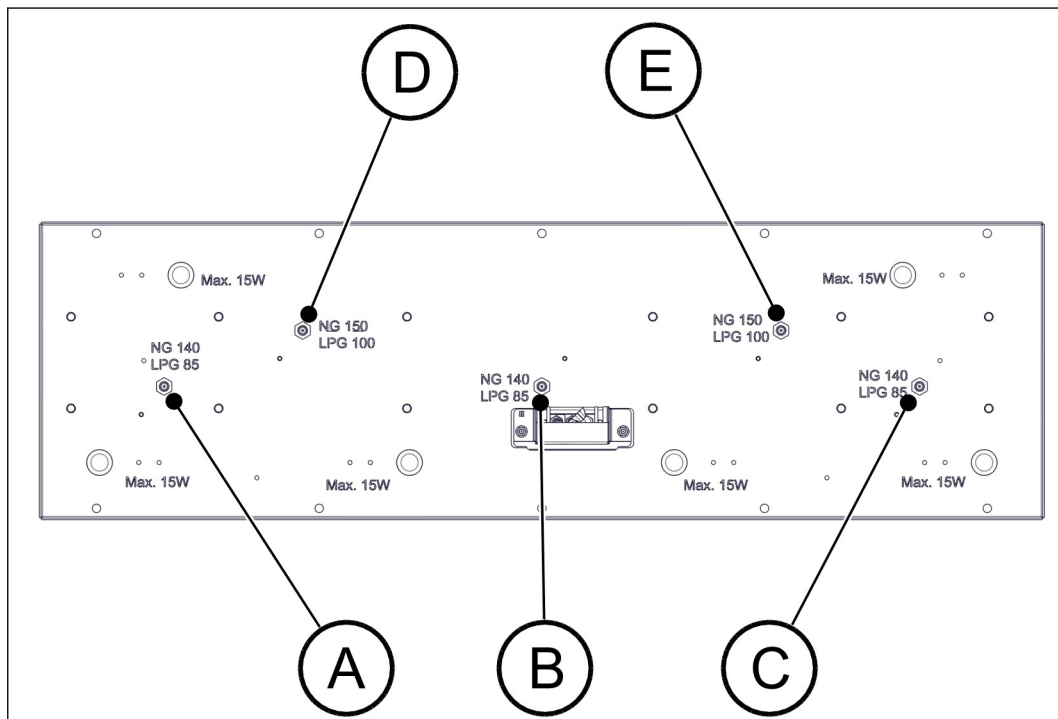
Figure 36. Position des entrées d'air primaires et des injecteurs de gaz
