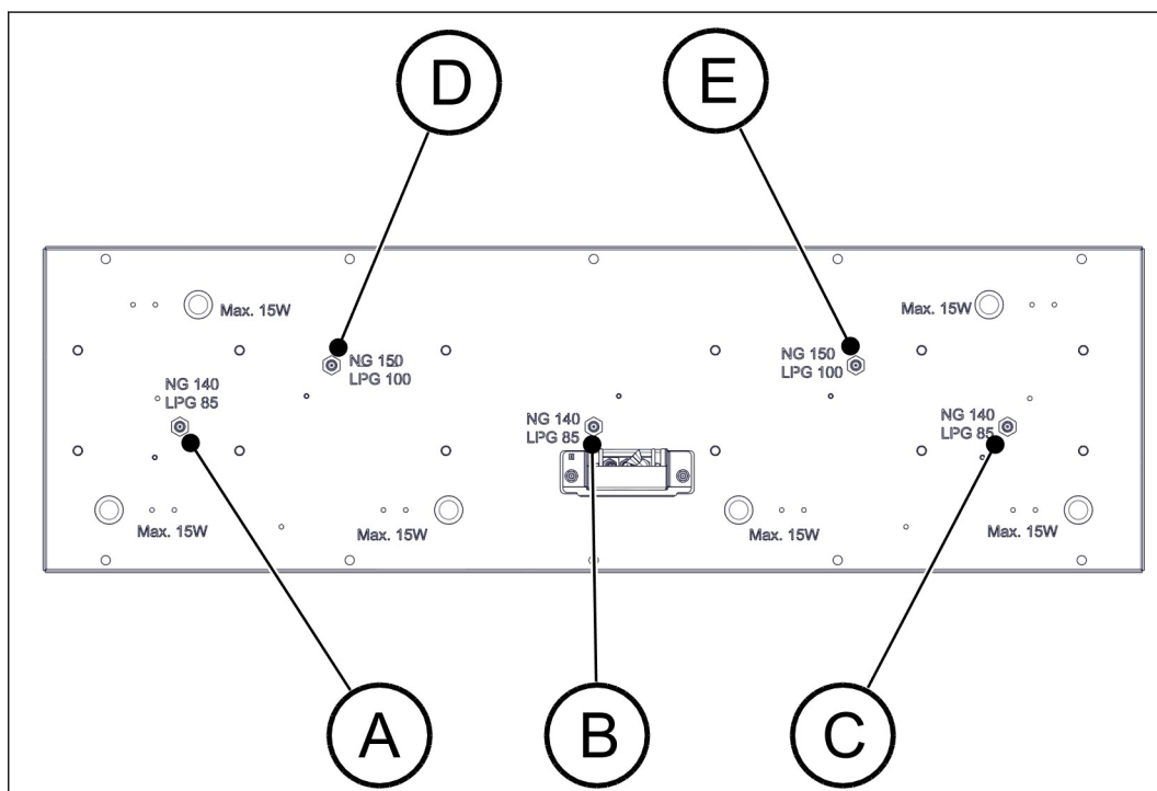
Figura 35. Posizioni degli ingressi dell'aria principali e degli iniettori di gas
