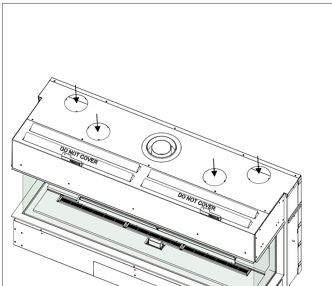
Figura 27. Posizione delle aperture di uscita dell'aria di convezione
