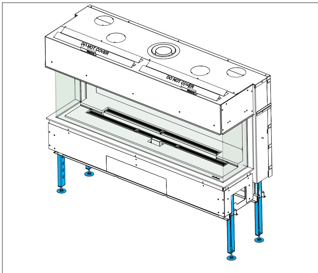
Figura 24. Allineare con le gambe ad altezza regolabile
