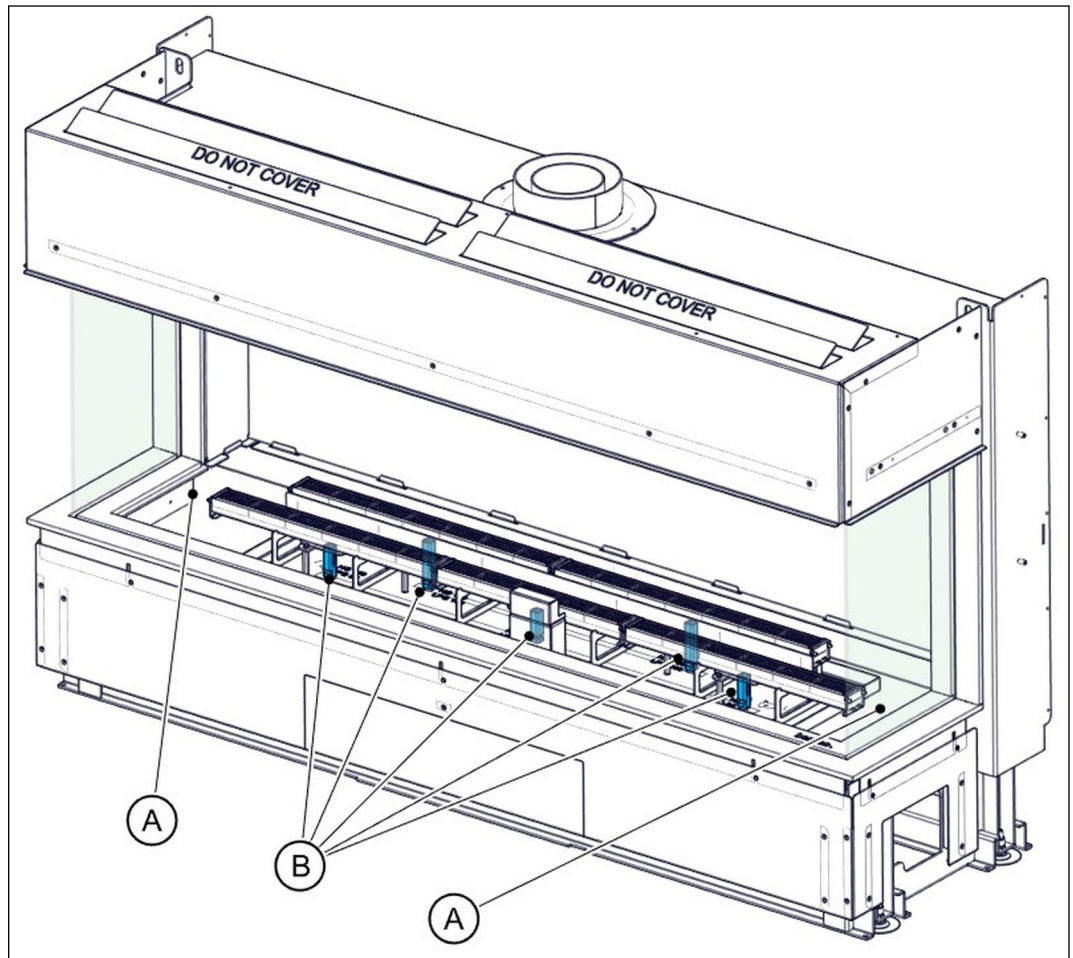
Figuur 32. Positie van luchtinlaat- en primaire luchtinlaatopeningen
