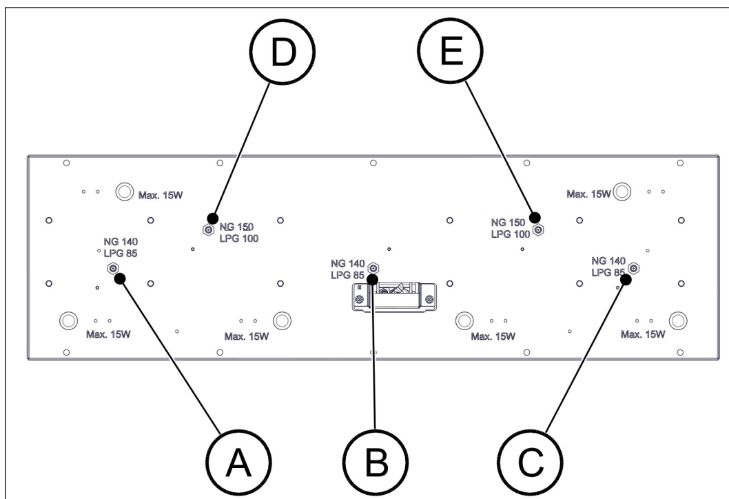
Figuur 36. Positie van primaire luchtinlaten en gasinjectoren
