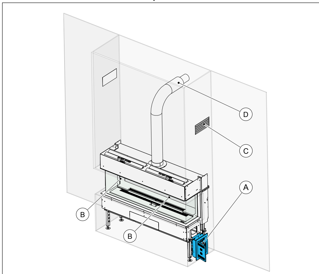
Figuur 9. Standaardinstallatie van een toestel zonder convectieset
