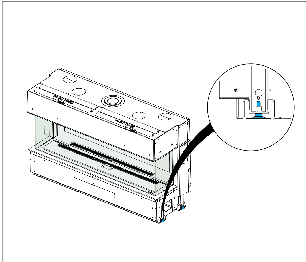
Figuur 23. Uitlijnen met behulp van stelvoeten
