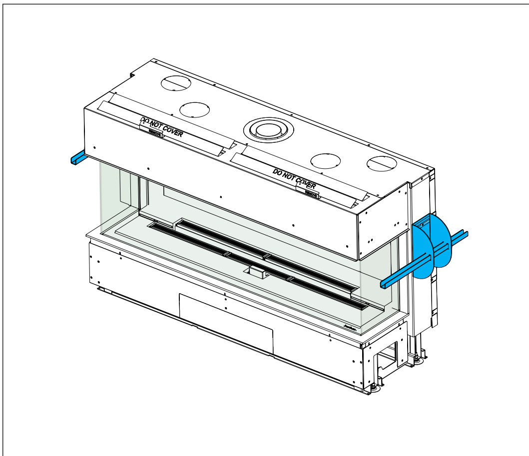
Figuur 22. Toestel met draaggrepen
