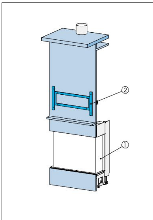
Abbildung 30. Installation eines Fernsehers über dem Gerät (Vorderansicht)
