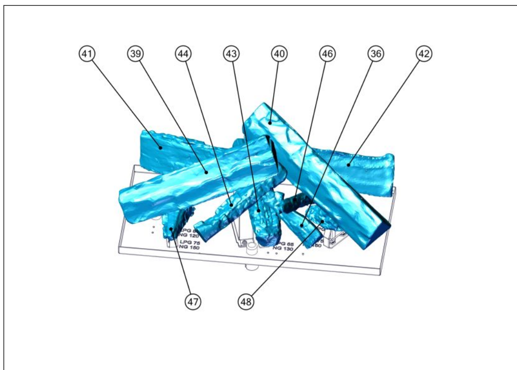
Abbildung 3. Überblick über den Keramikholzscheitsatz
