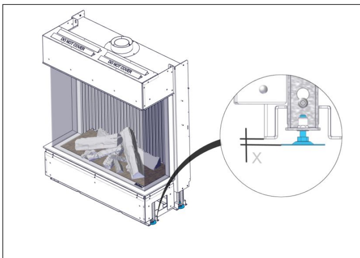
Figura 23. Alineación con los pies ajustables
