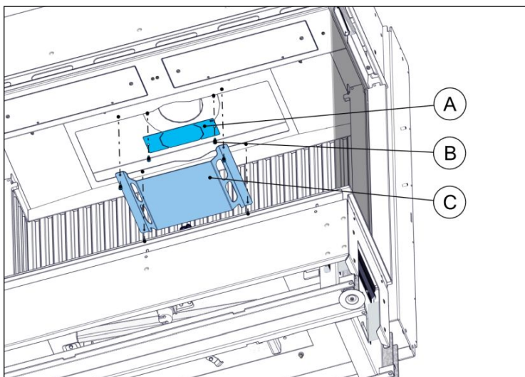
Figura 29. Placa de restricción y desviadora
