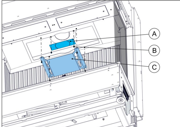
Abbildung 29. Begrenzerplatte und Umlenkplatte
