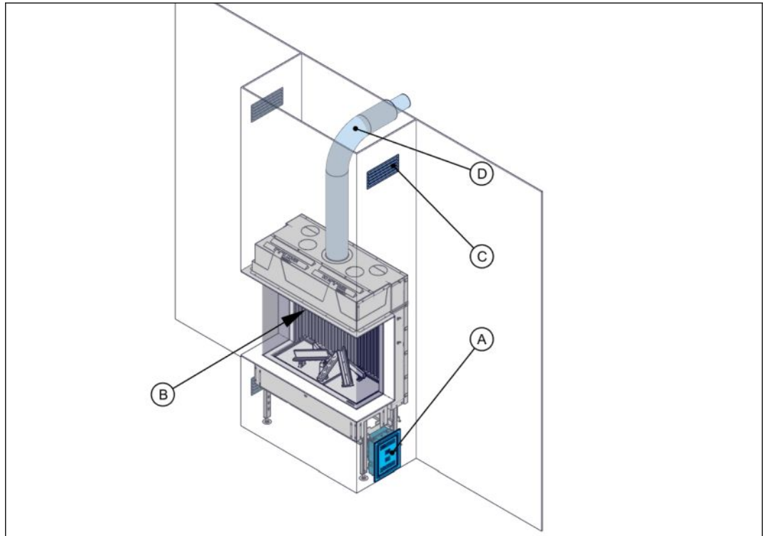
Abbildung 9. Typische Installation eines Geräts ohne Konvektionssatz
