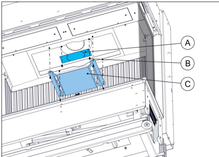
Figura 29. Piastra di restrizione e pannello deflettore
