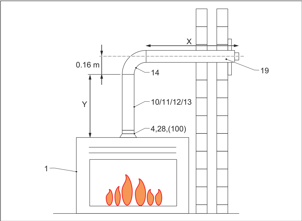
Systèmes de canalisations concentriques rigides
