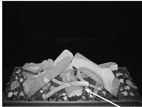
Position der Zündflamme
