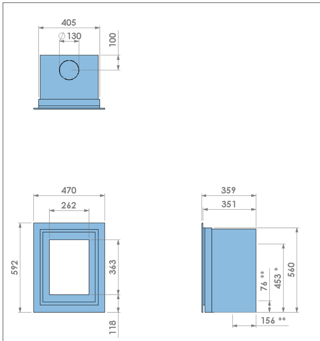
Abbildung 16. Abmessungen des Geräts mit klassischem Rahmen und Tür mit Stahlrahmen
