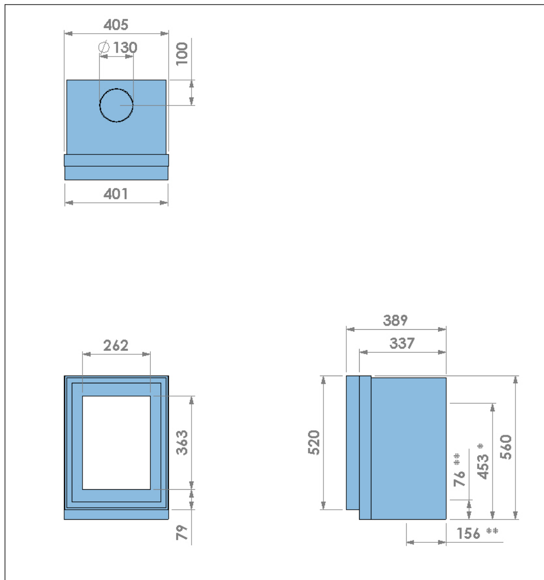
Abbildung 14. Abmessungen des Geräts mit Einbaurahmen und Tür mit Stahlrahmen
