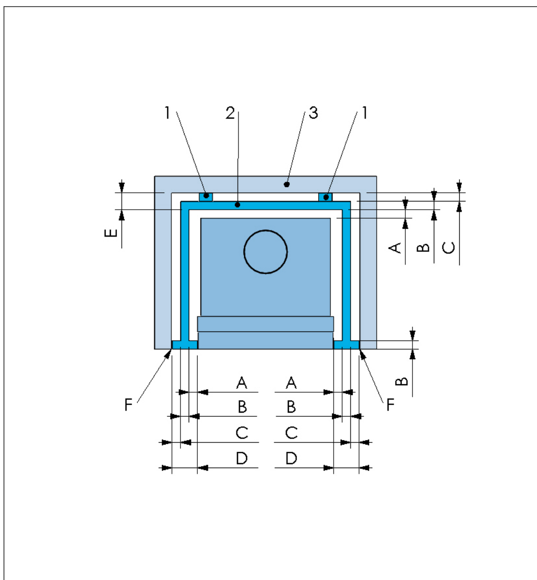
Figuur 7. Afstanden tot niet-brandbare wand – Boven aanzicht
