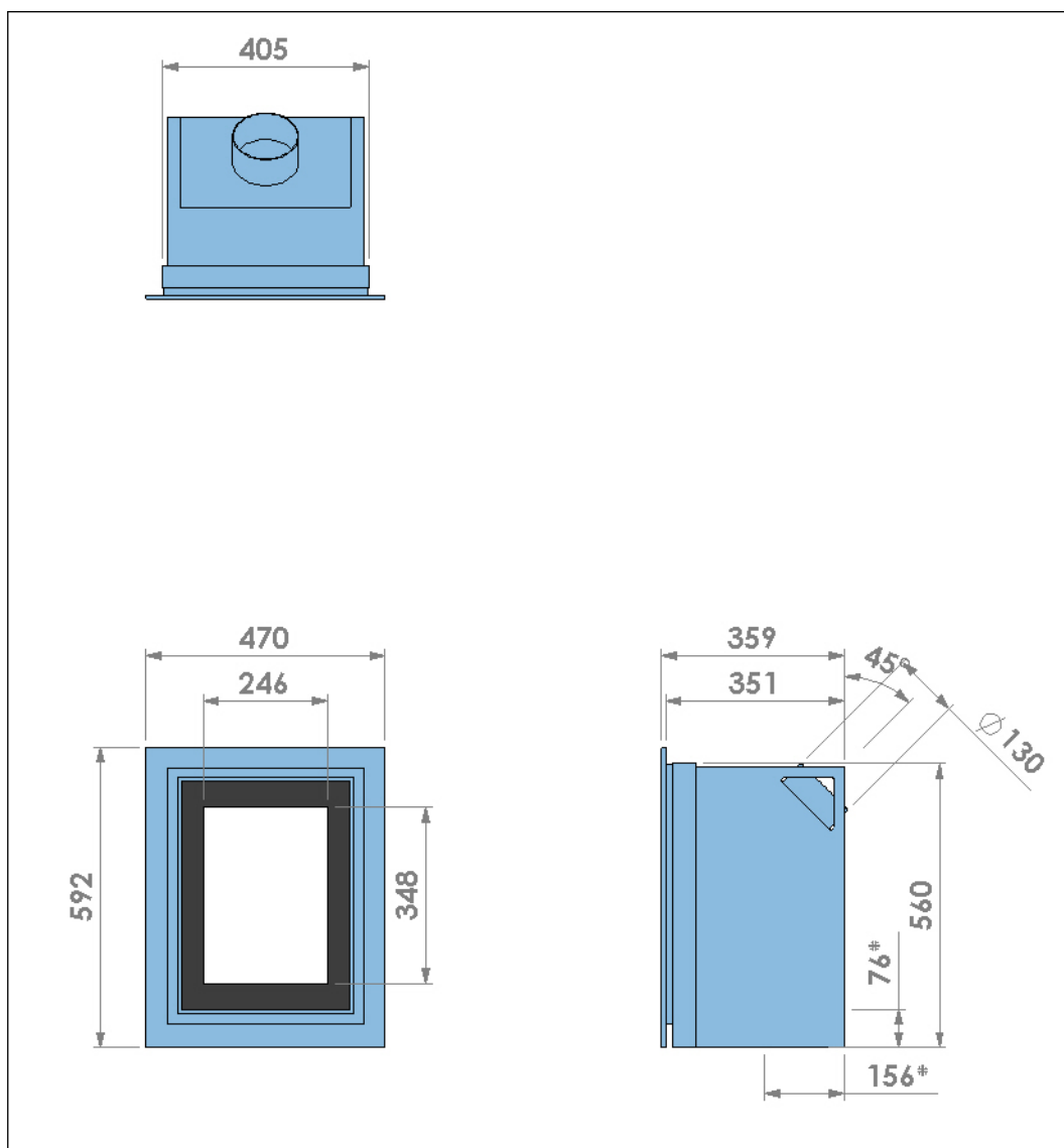
Figuur 17. Afmetingen van een toestel met een klassiek kader, een 45° rookkanaalconnector en een deur van gescreend glas
