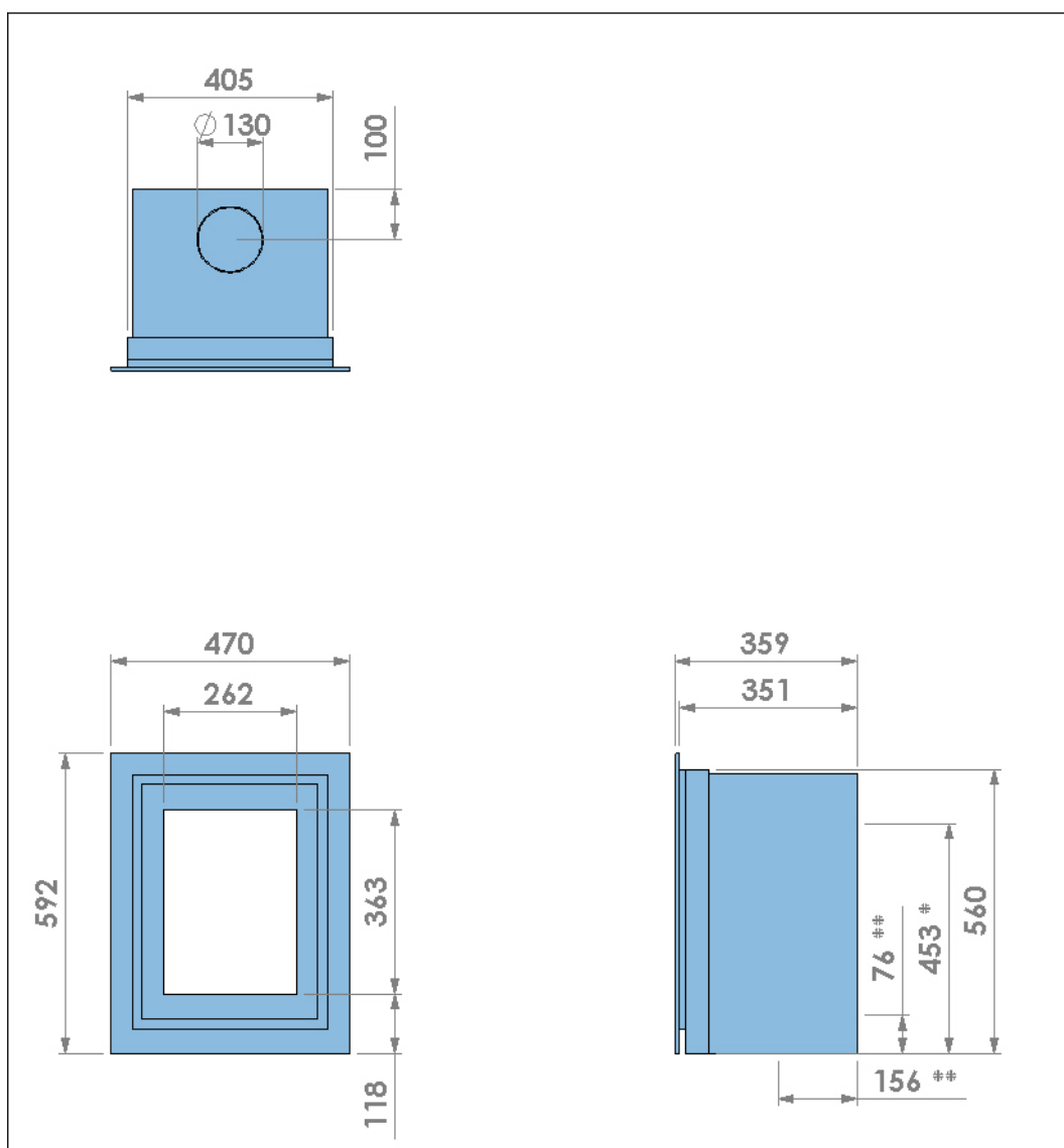
Figuur 16. Afmetingen van een toestel met een klassiek kader en een deur in een metalen kader
