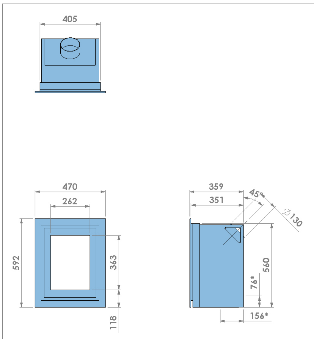
Figuur 18. Afmetingen van een toestel met een klassiek kader, een 45° rookkanaalconnector en een deur in een metalen kader
