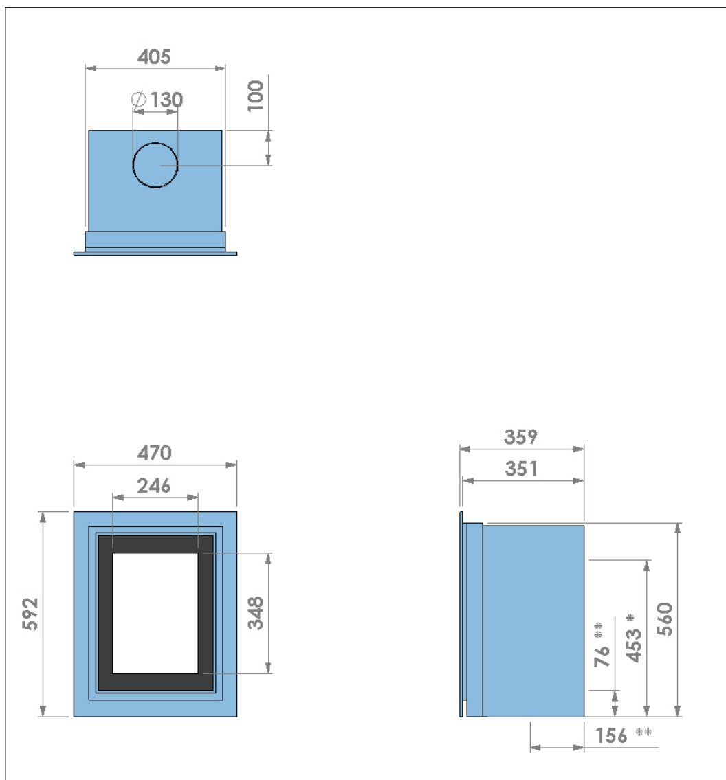
Figuur 15. Afmetingen van een toestel met een klassiek kader en een deur van gescreend glas
