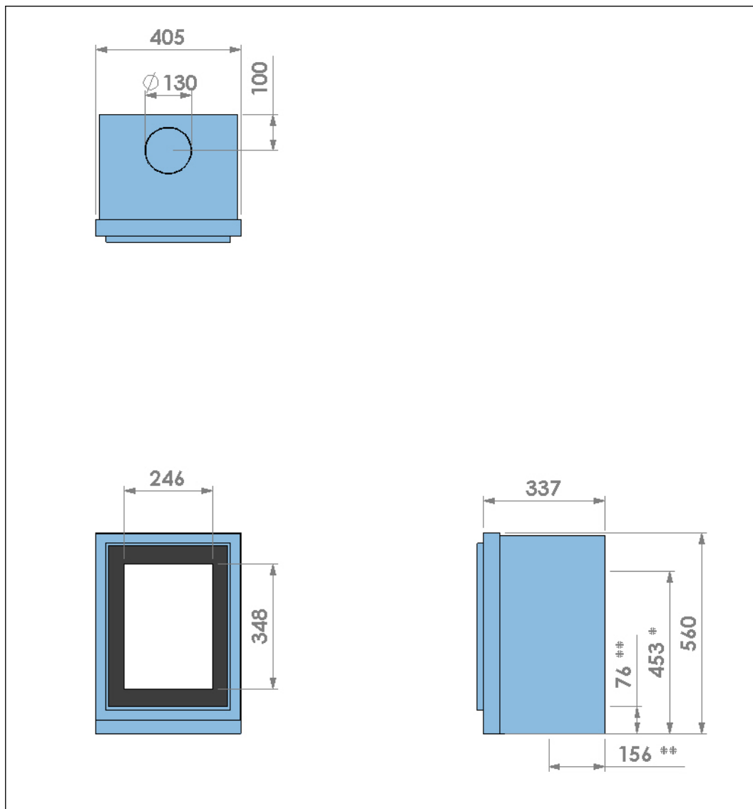
Figuur 11. Afmetingen van een kaderloos toestel met een deur van gescreend glas
