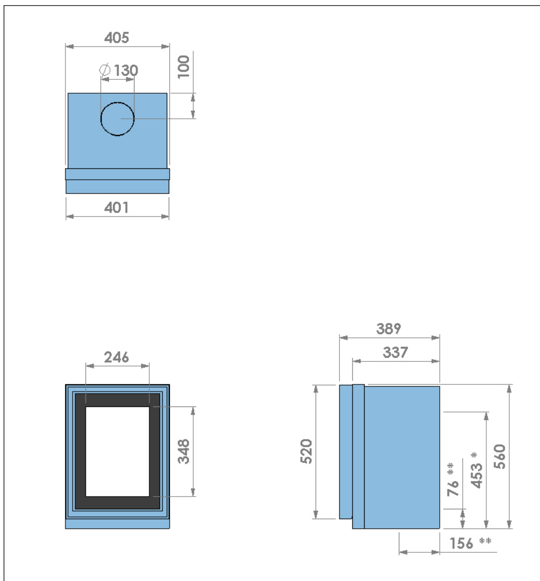
Figuur 13. Afmetingen van een toestel met een inbouwkader en een deur van gescreend glas
