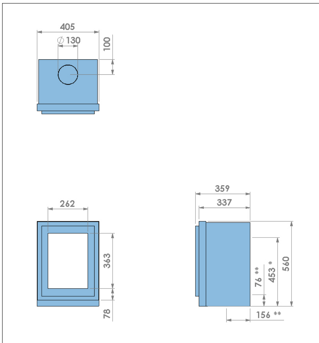
Figuur 12. Afmetingen van een kaderloos toestel met een deur in een stalen kader
