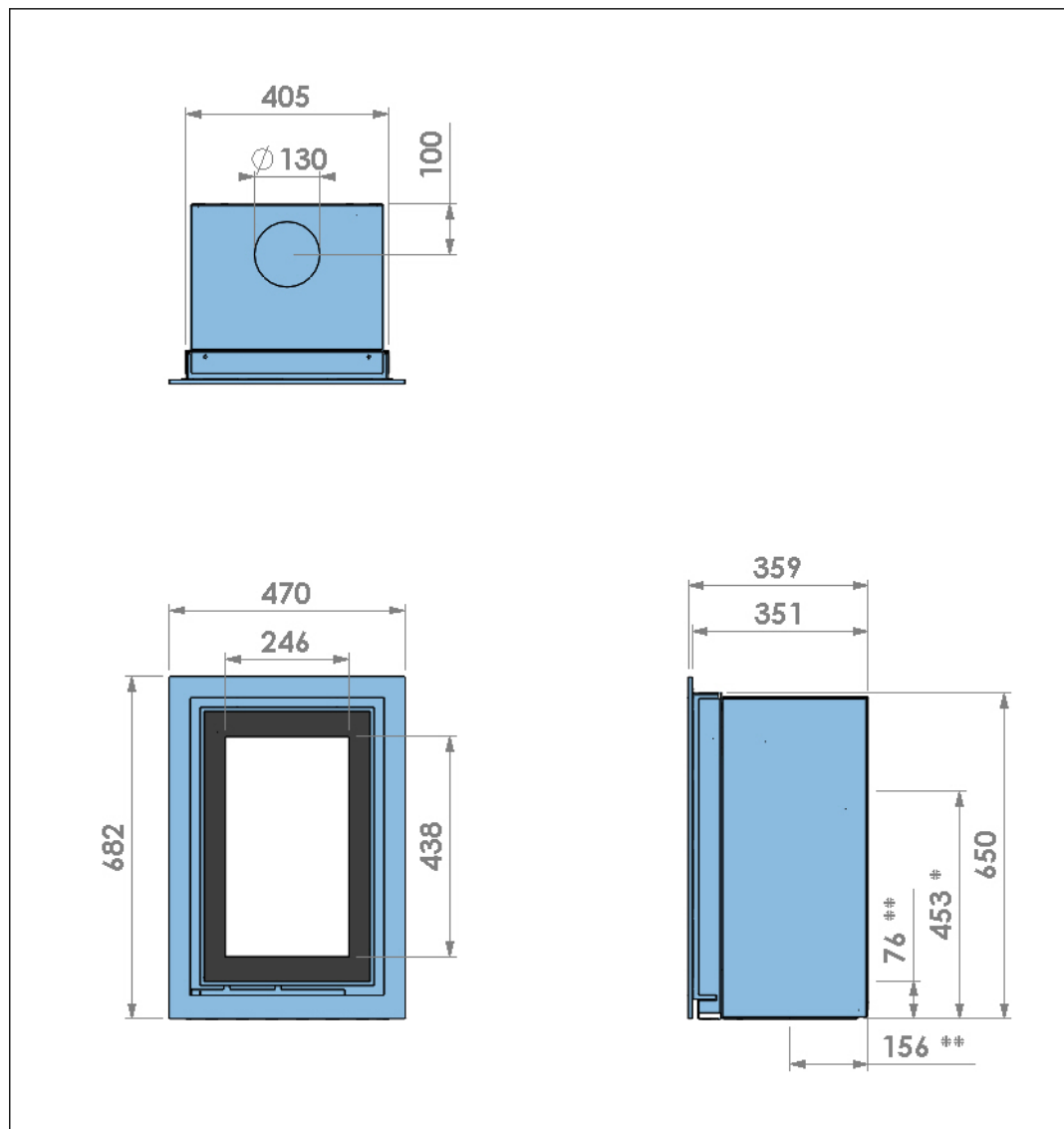
Abbildung 15. Abmessungen des Geräts mit klassischem Rahmen und abgeschirmter Glastür
