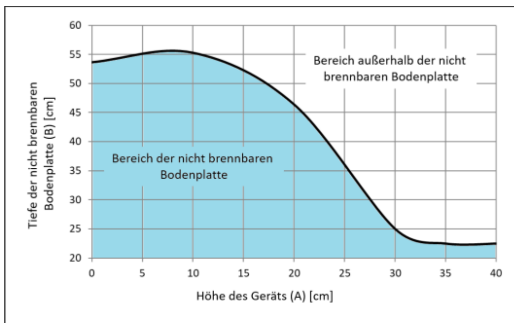
Abbildung 8. Höhe des Geräts im Vergleich zur Tiefe der feuerfesten Bodenplatte
