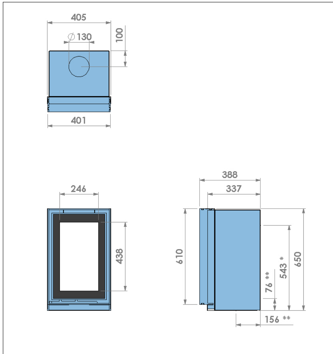
Abbildung 13. Abmessungen des Geräts mit Einbaurahmen und abgeschirmter Glastür
