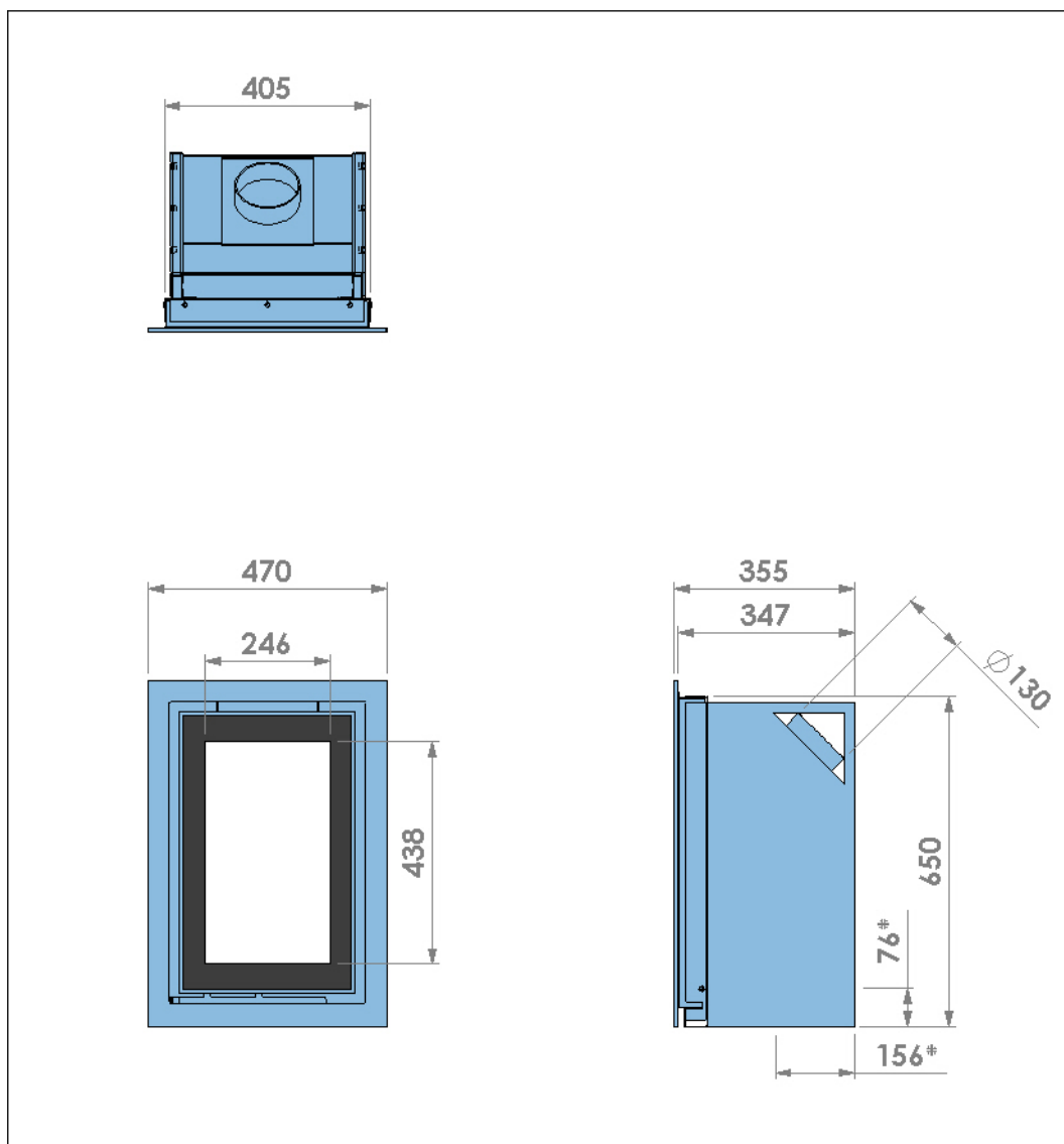
Abbildung 17. Abmessungen des Geräts mit klassischem Rahmen, 45°-Abzugsanschluss und abgeschirmter Glastür
