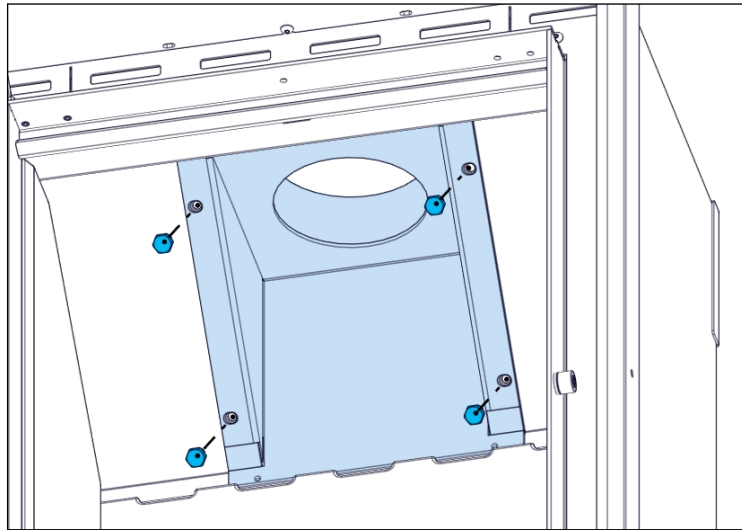
Abbildung 10. Abzugsrohranschluss
