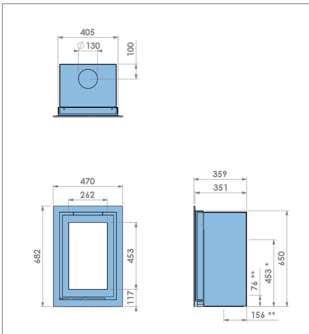
Abbildung 16. Abmessungen des Geräts mit klassischem Rahmen und Tür mit Stahlrahmen
