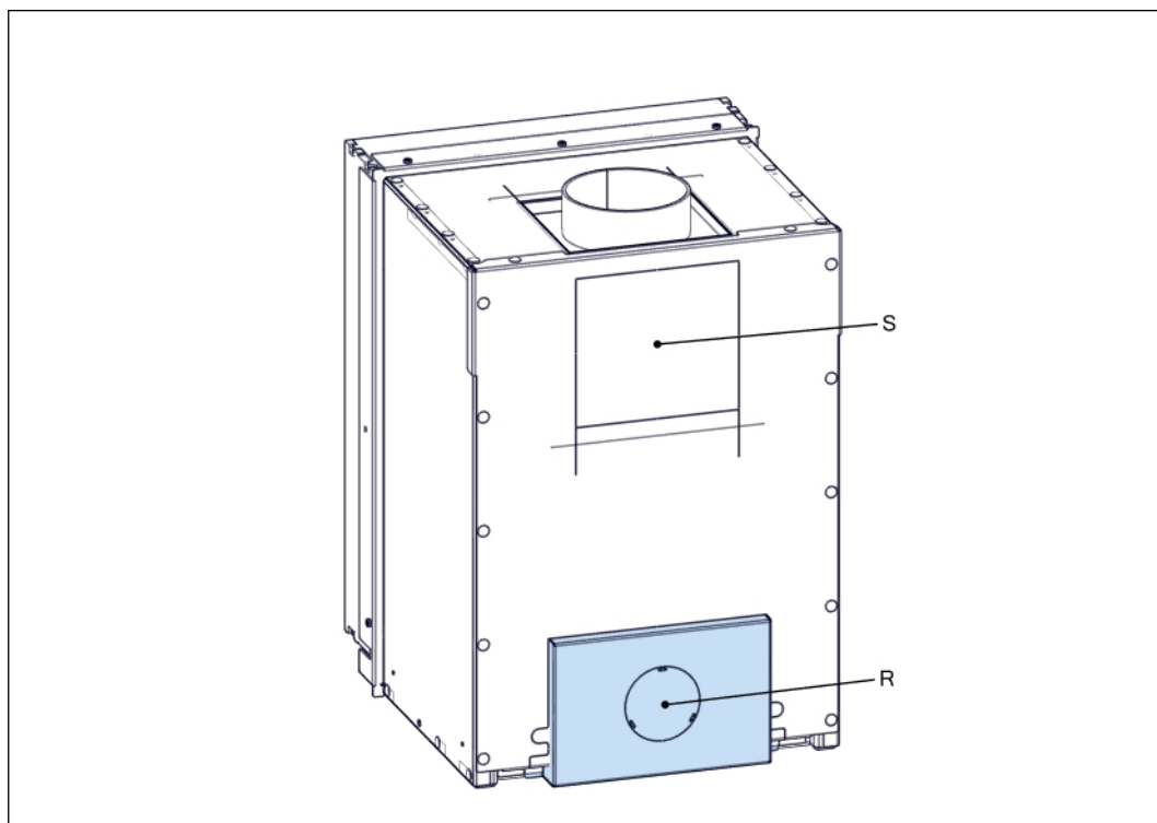
Abbildung 2. Untersicht der Unilux-7 45 mit abgeschirmter Tür
