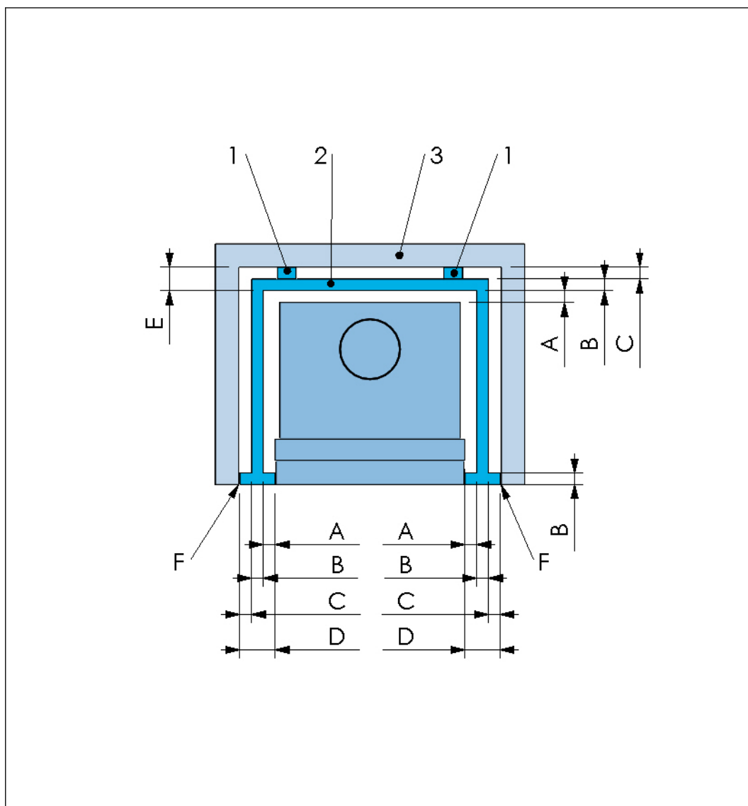
Abbildung 6. Abstände zur brennbaren Wand – Draufsicht
