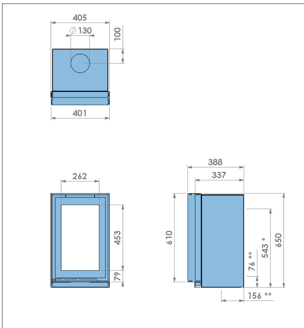
Abbildung 14. Abmessungen des Geräts mit Einbaurahmen und Tür mit Stahlrahmen
