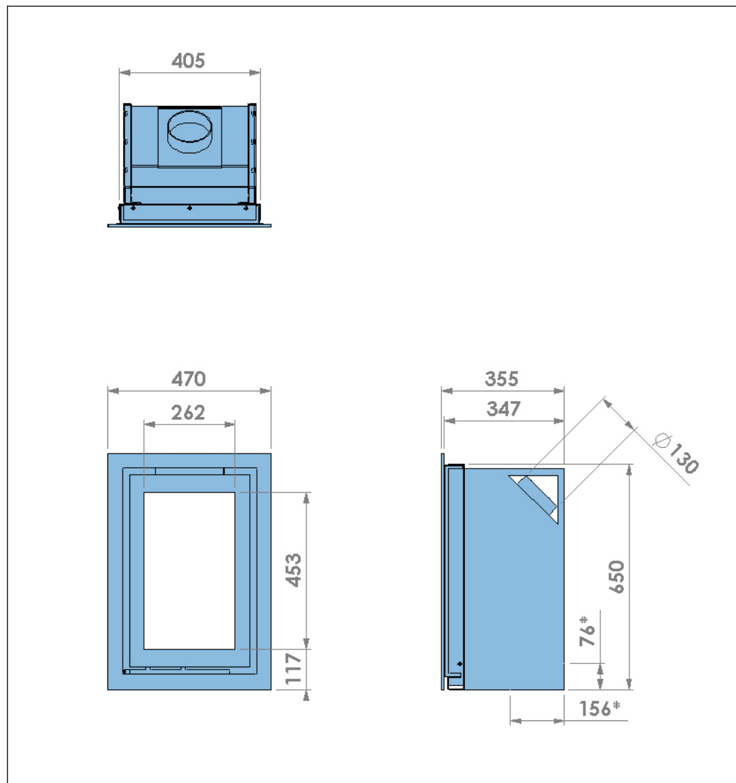
Abbildung 18. Abmessungen des Geräts mit klassischem Rahmen, 45°-Abzugsanschluss und Tür mit Stahlrahmen
