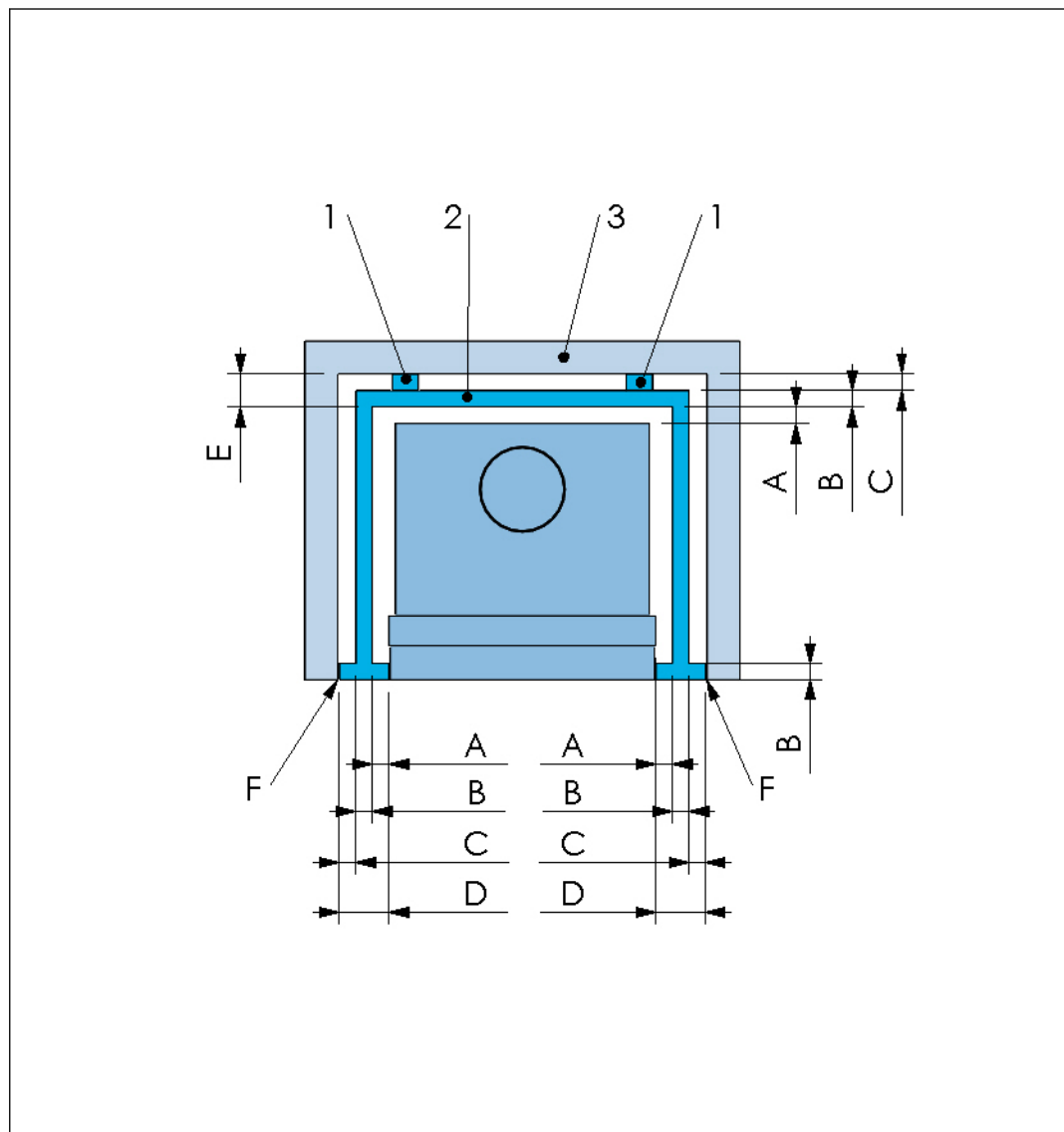
Abbildung 7. Abstände zu nicht brennbarer Wand – Draufsicht
