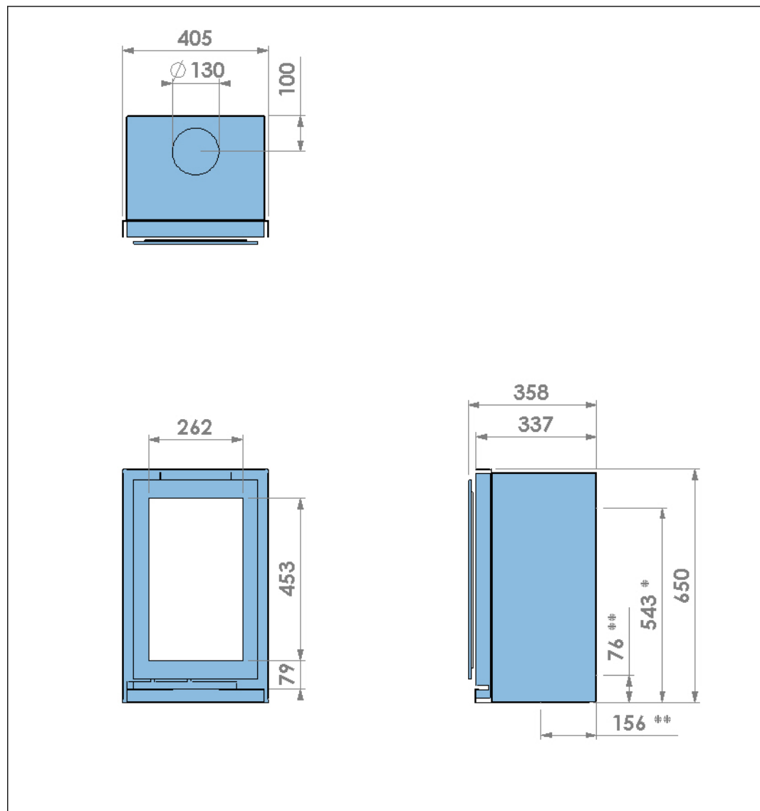
Abbildung 12. Abmessungen der rahmenlosen Vorrichtung mit Tür mit Stahlrahmen
