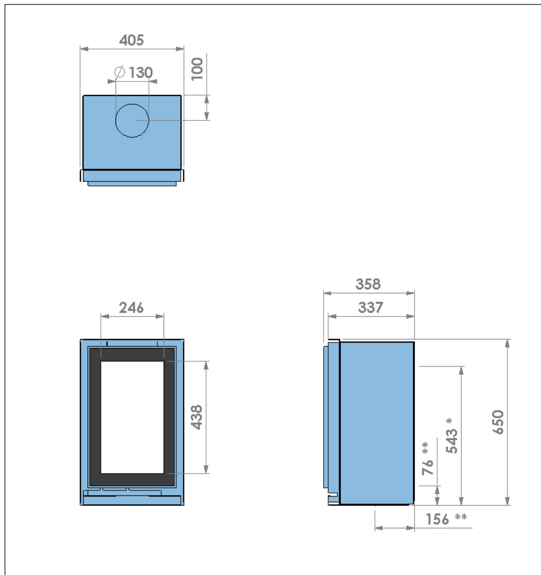
Abbildung 11. Abmessungen der rahmenlosen Vorrichtung mit abgeschirmter Glastür
