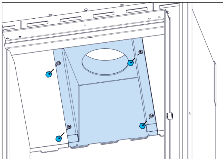
Figuur 10. Rookkanaalpijpconnector
