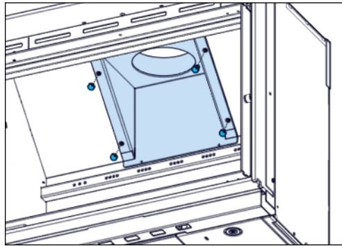
Abbildung 11. Abzugsrohranschluss
