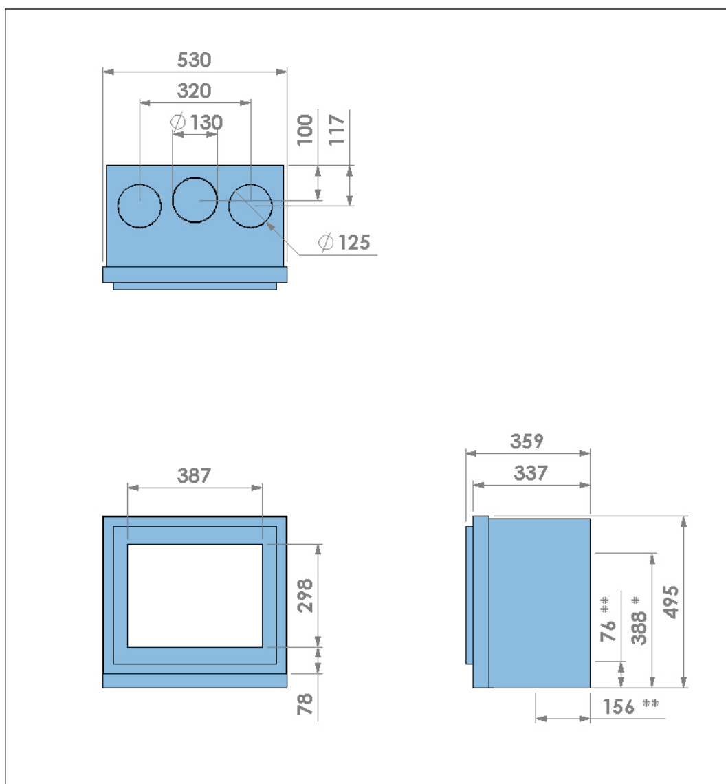
Abbildung 13. Abmessungen der rahmenlosen Vorrichtung mit Tür mit Stahlrahmen
