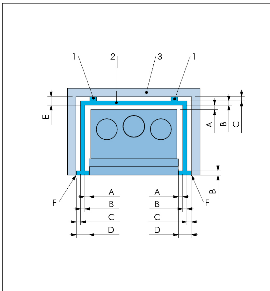
Figure 8. Dégagements avec paroi inflammable - Vue du dessus
