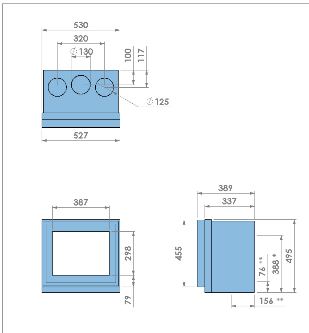
Figuur 15. Afmetingen van een toestel met een inbouwkader en een deur in een metalen kader
