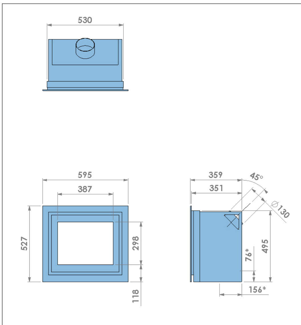
Figuur 19. Afmetingen van een toestel met een klassiek kader, een 45° rookkanaalconnector en een deur in een metalen kader
