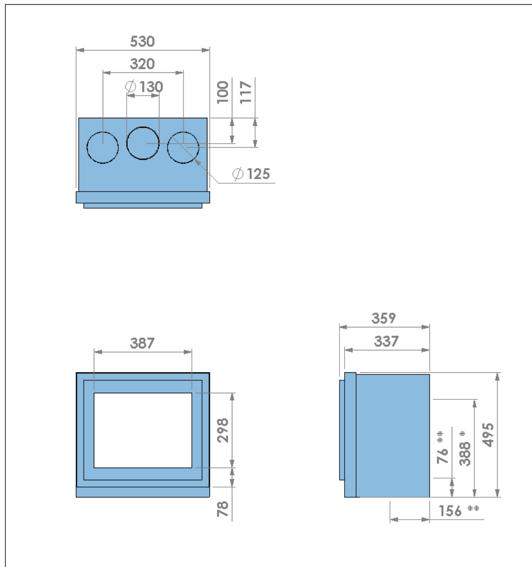
Figuur 13. Afmetingen van een kaderloos toestel met een deur in een stalen kader
