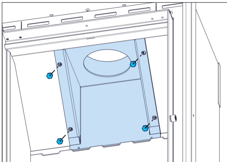
Figure 11. Connecteur de tuyau de conduit
