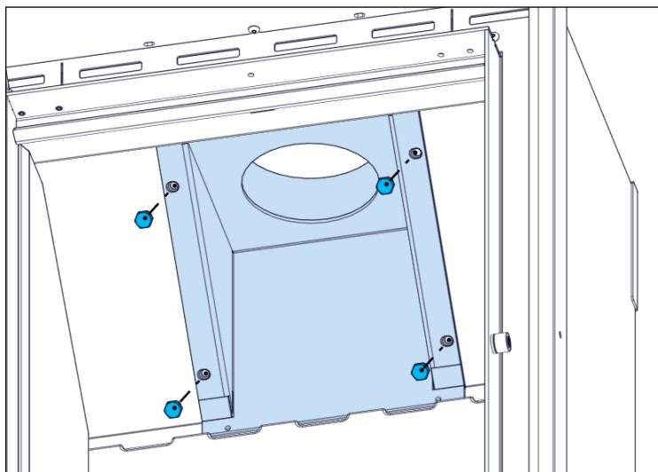
Figuur 11. Rookkanaalpijpconnector
