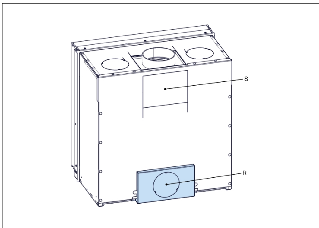
Figuur 3. Achteraanzicht van de Unilux-7 67
