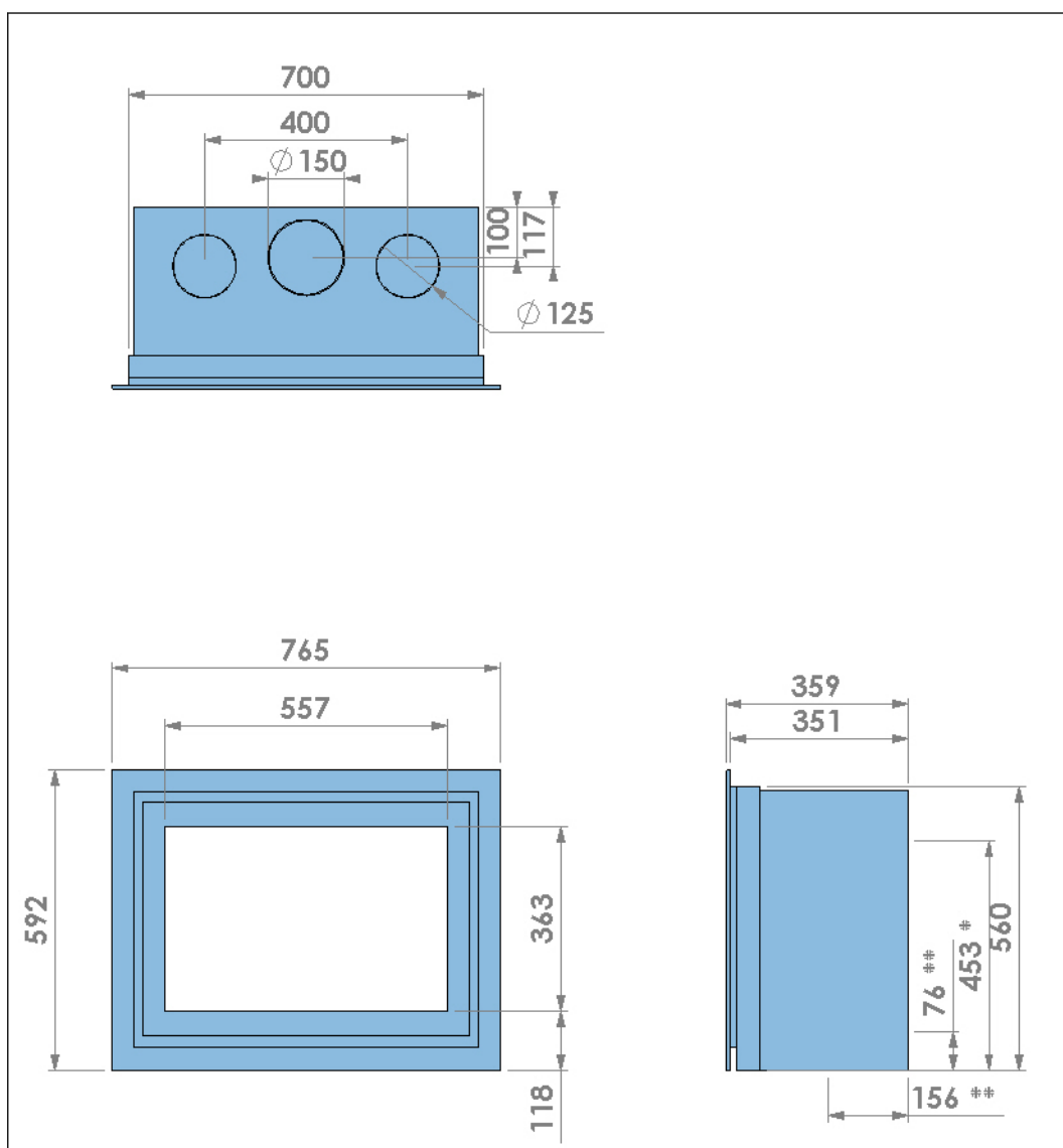
Figure 17. Dimensions d'appareil avec châssis classique et porte à châssis en métal
