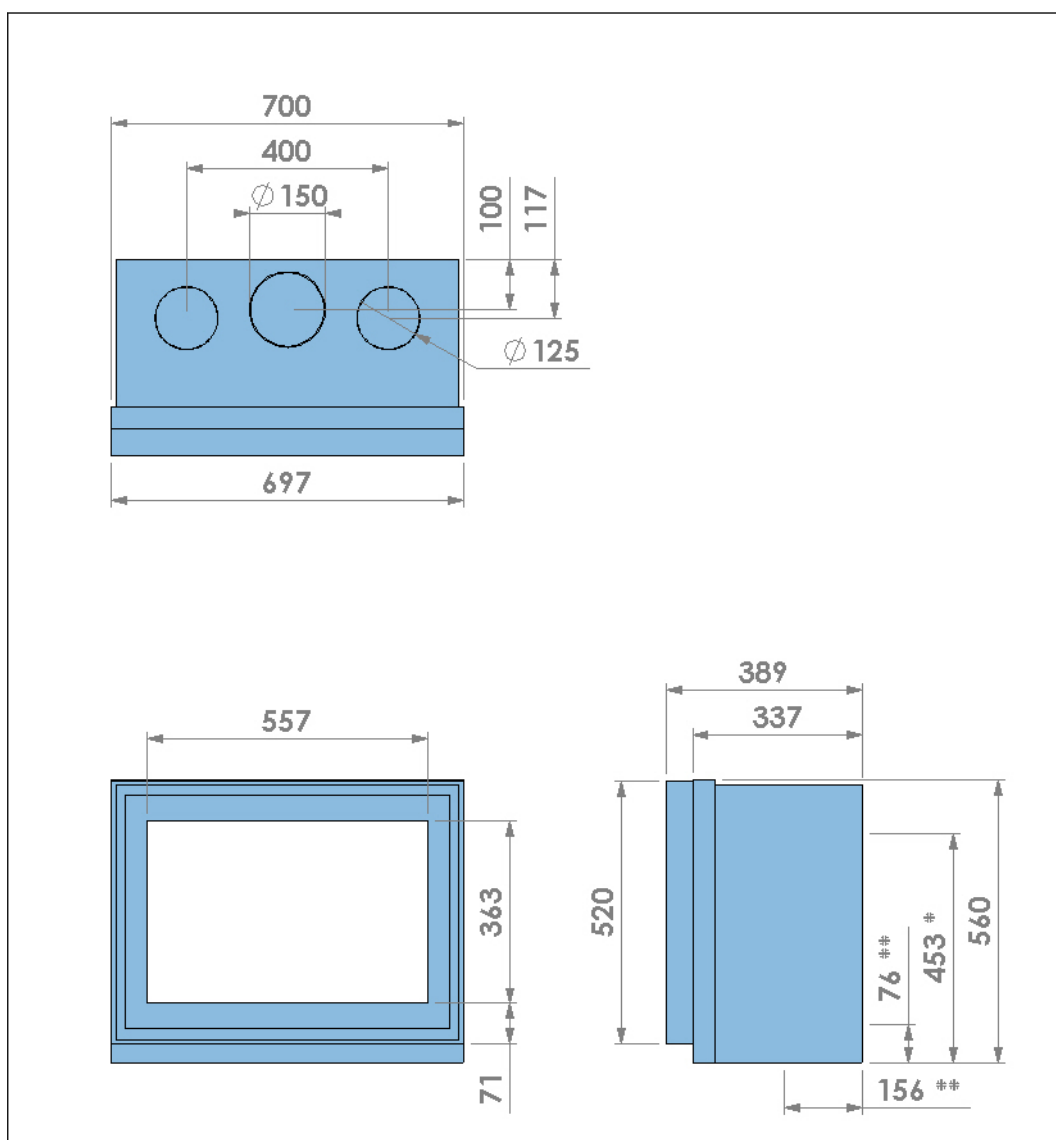
Figure 15. Dimensions d'appareil avec châssis intégré et porte à châssis en métal
