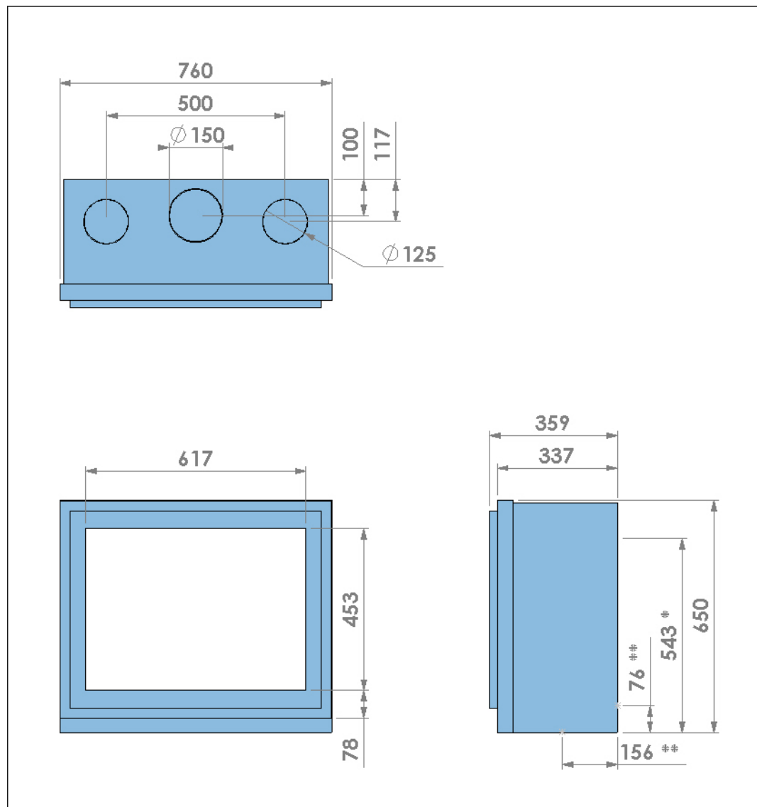
Abbildung 13. Abmessungen des Geräts mit Tür mit Stahlrahmen
