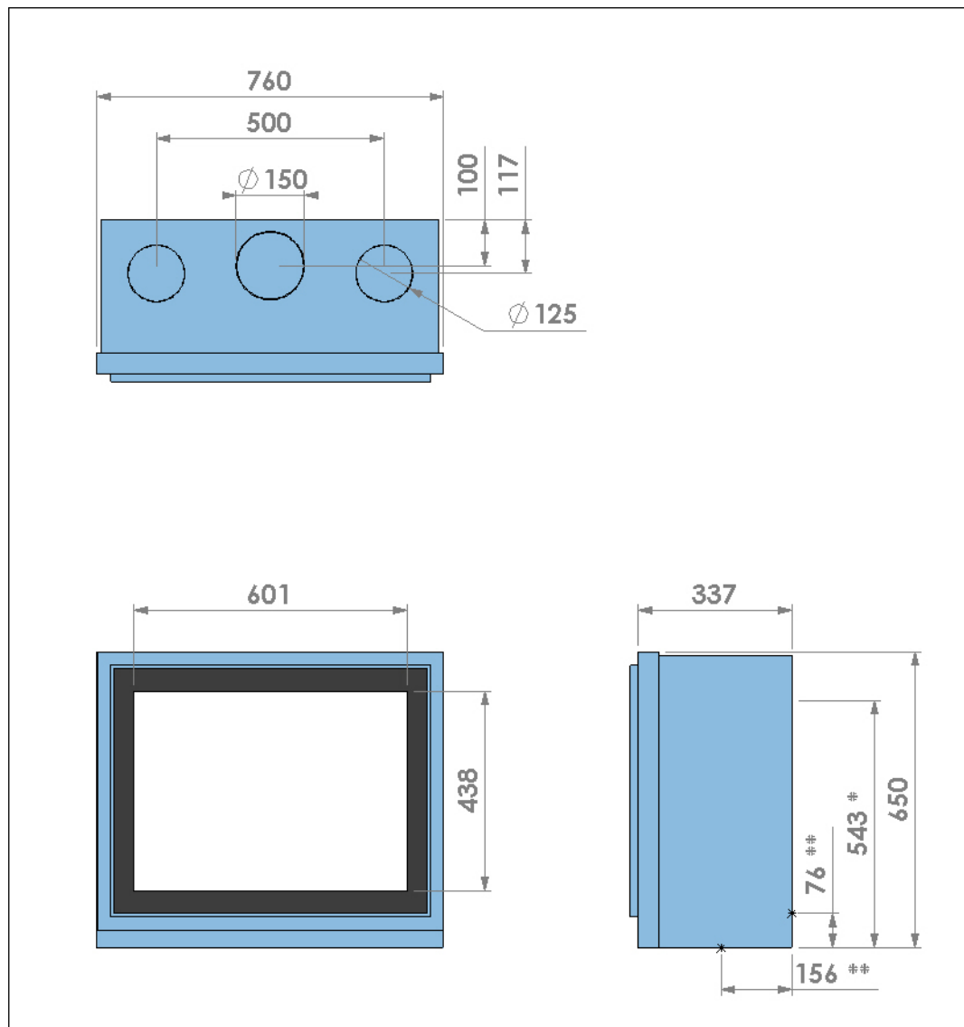
Abbildung 12. Abmessungen des Geräts mit abgeschirmter Glastür
