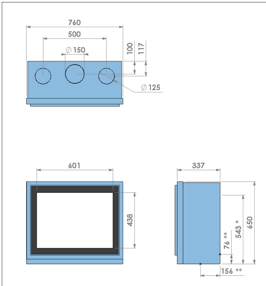
Figure 12. Dimensions d'appareil avec porte à vitre blindée
