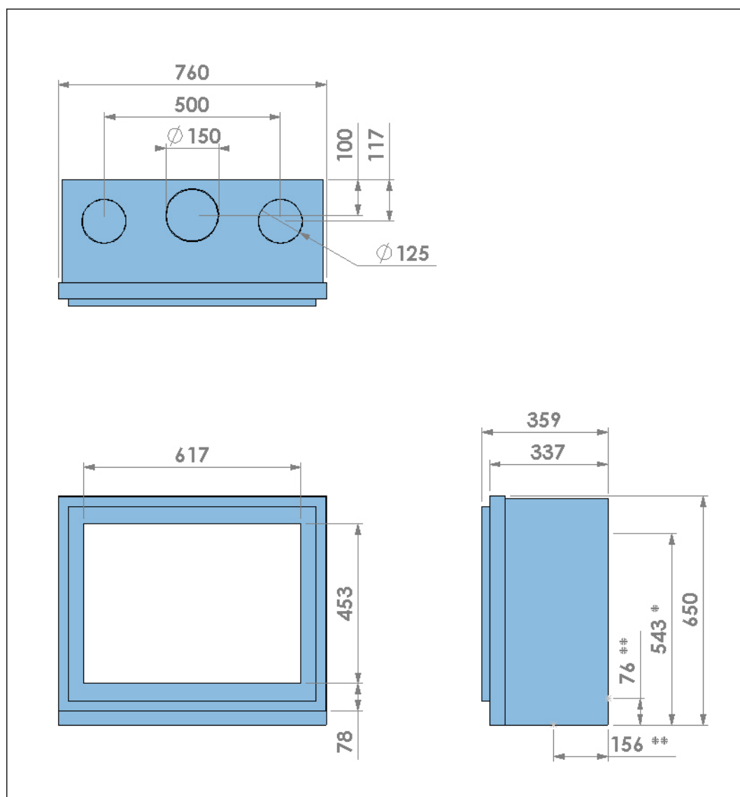
Figure 13. Dimensions d'appareil avec porte à châssis en acier
