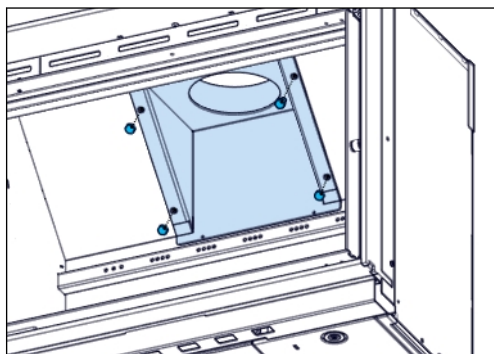
Figure 11. Connecteur de tuyau de conduit
