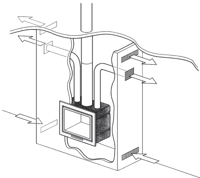
Abbildung 2: Anwendung Konvektionsset und Ventilation Feuerstelle (schematisch)
